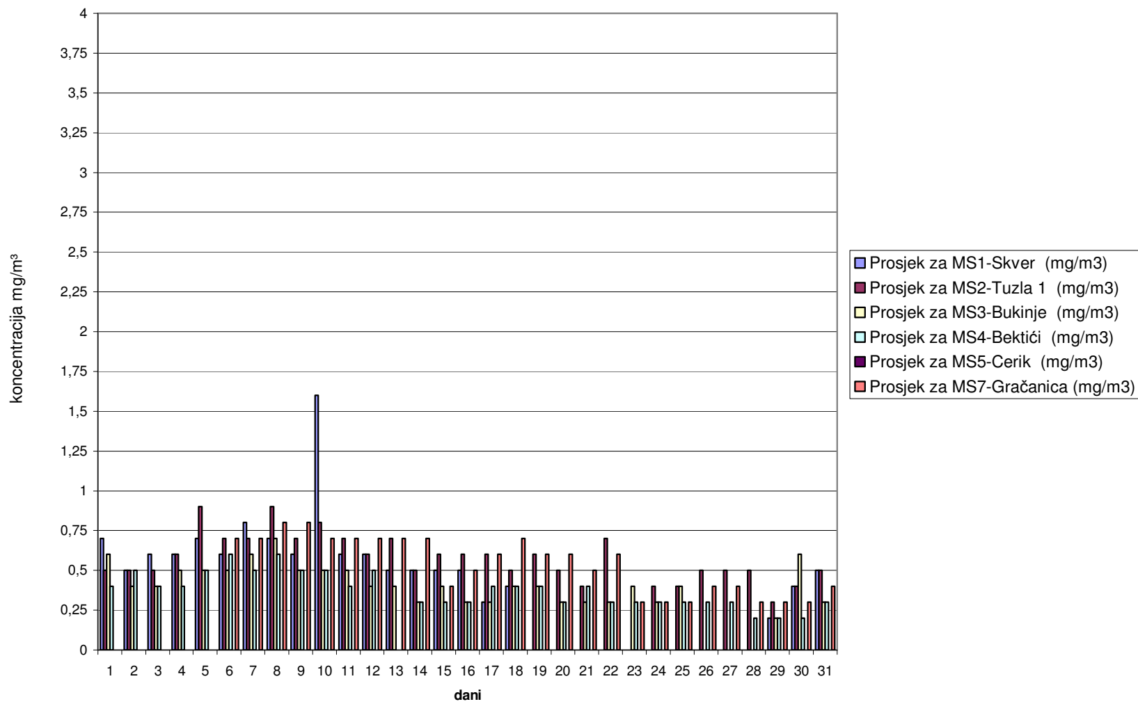
Slika 3. Grafički prikaz prosječnih dnevnih vrijednosti ugljenmonoksida (CO) za mjesec maj 2006. godine
