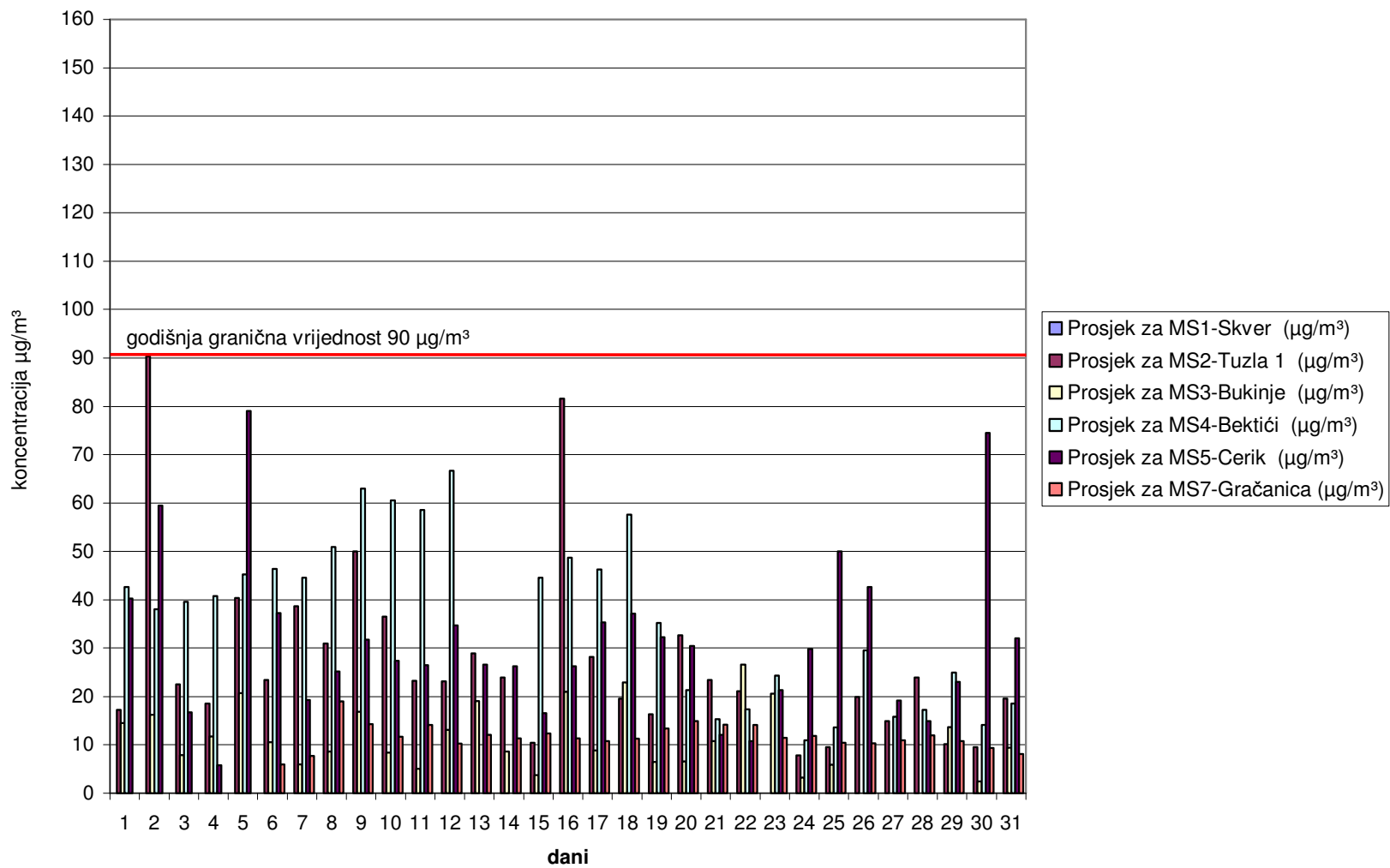
Slika 1. Grafički prikaz prosječnih dnevnih vrijednosti sumpordioksida (SO 2 ) za mjesec maj 2006. godine
