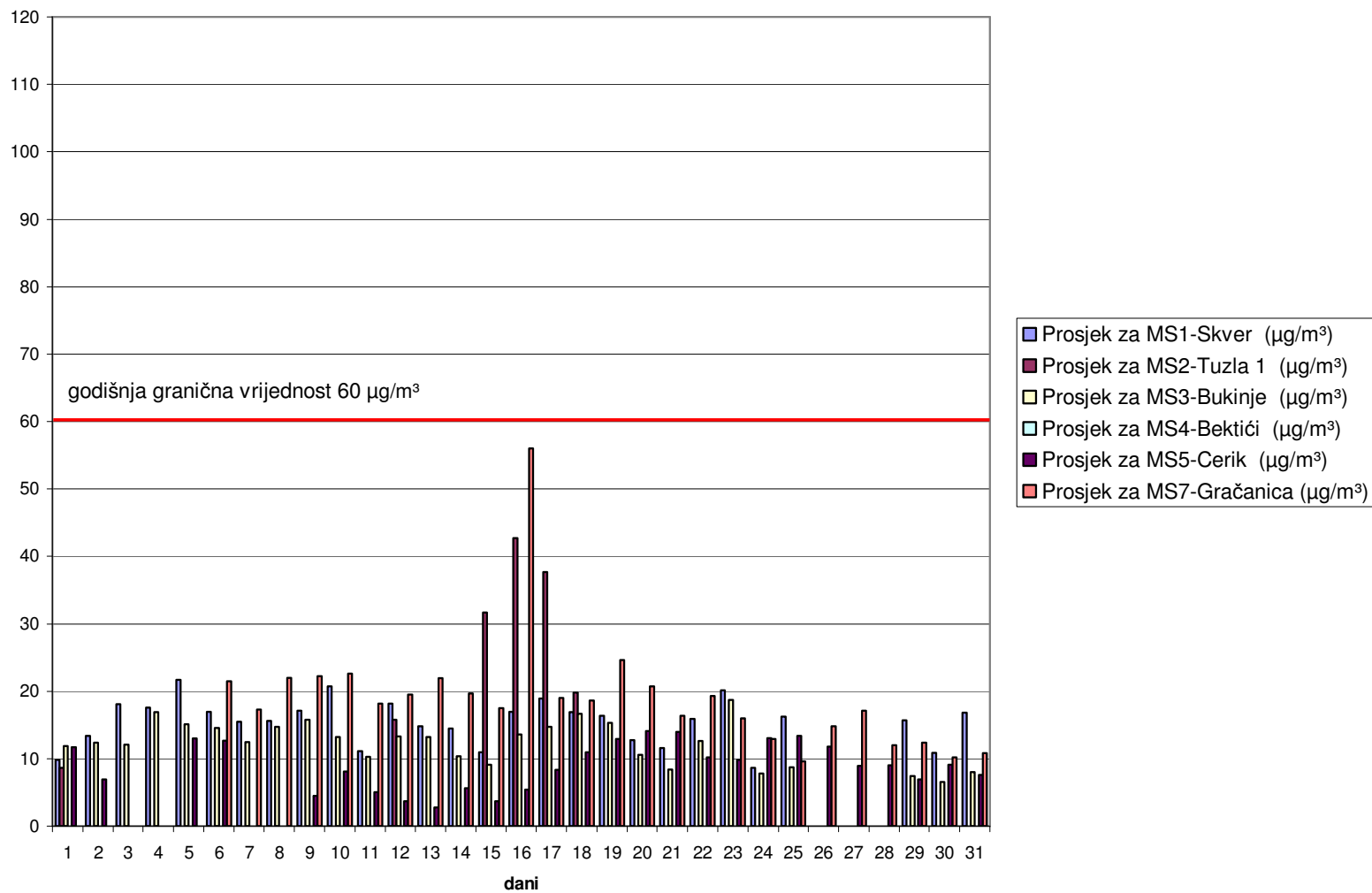
Slika 2. Grafički prikaz prosječnih dnevnih vrijednosti azotdioksida (NO 2 ) za mjesec maj 2006. godine
