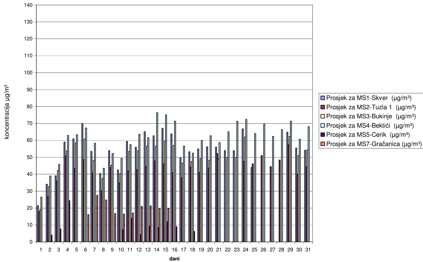
Slika 4. Grafički prikaz prosječnih dnevnih vrijednosti ozona ( O_3 ) za mjesec maj 2006. godine
