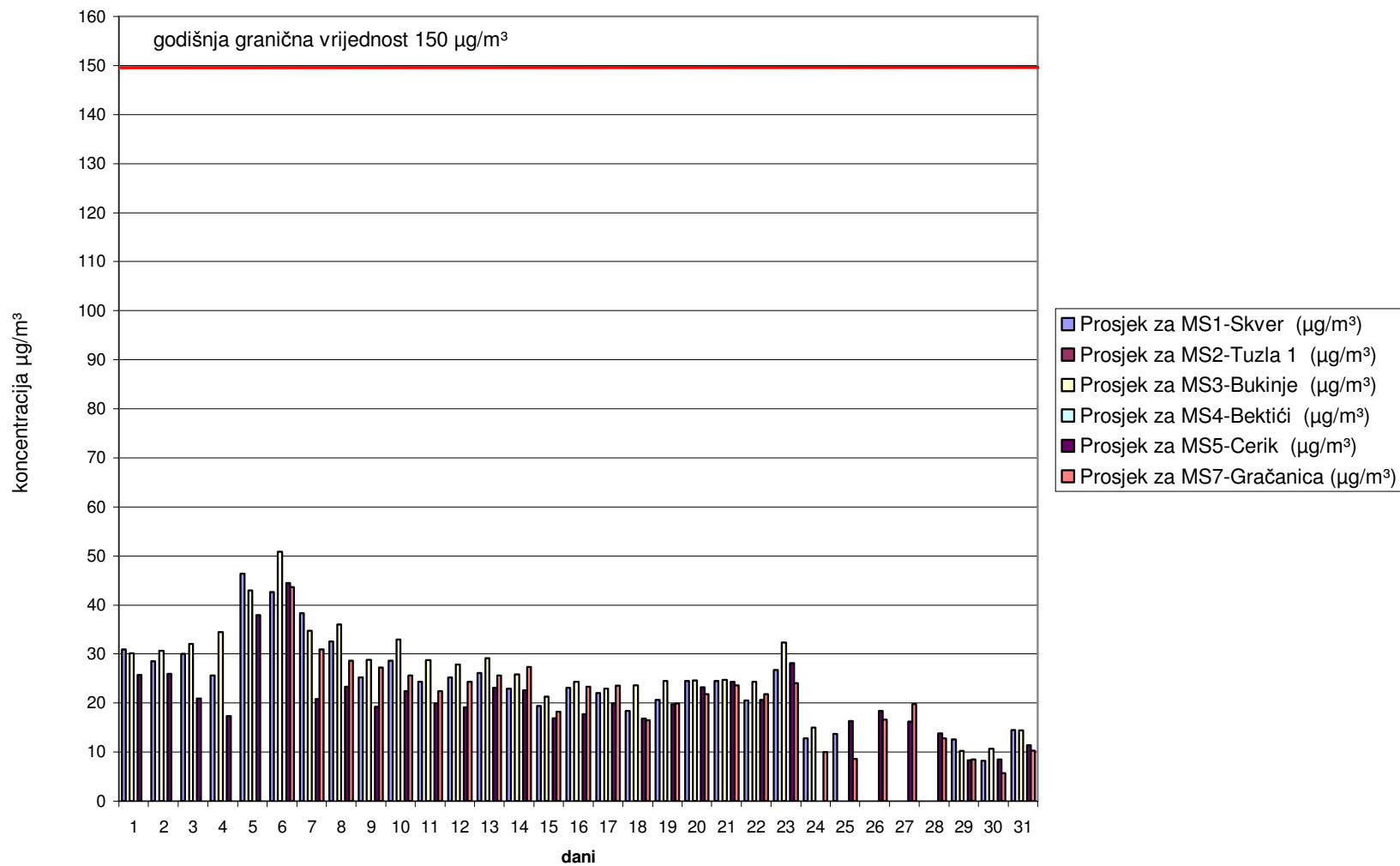
Slika 5. Grafički prikaz prosječnih dnevnih vrijednosti prašine ( \text{PM}_{2.5} ) za mjesec maj 2006. godine
