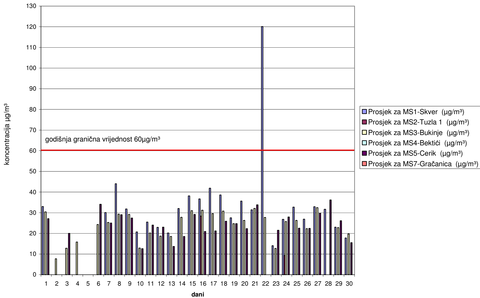
Slika 2. Grafički prikaz prosječnih dnevnih vrijednosti azotdioksida (NO 2 ) za mjesec novembar/studeni 2006. godine
