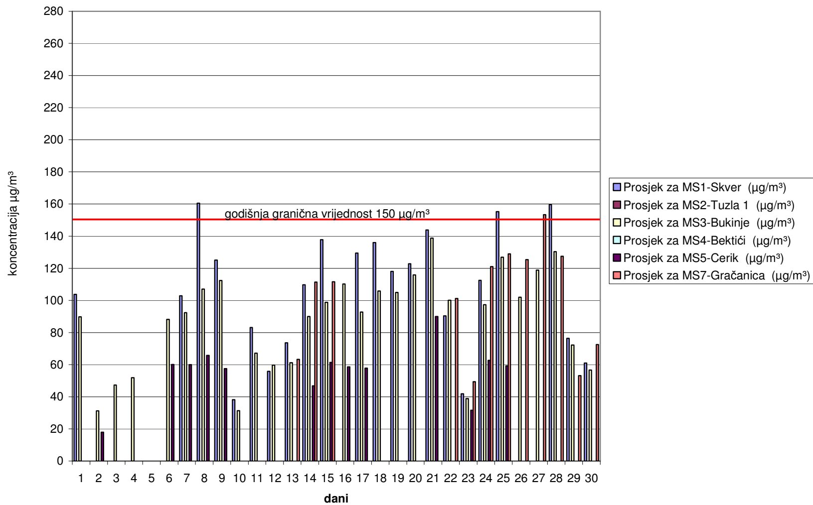
Slika 5. Grafički prikaz prosječnih dnevnih vrijednosti prašine (PM 2.5 ) za mjesec novembar/studeni 2006. godine
