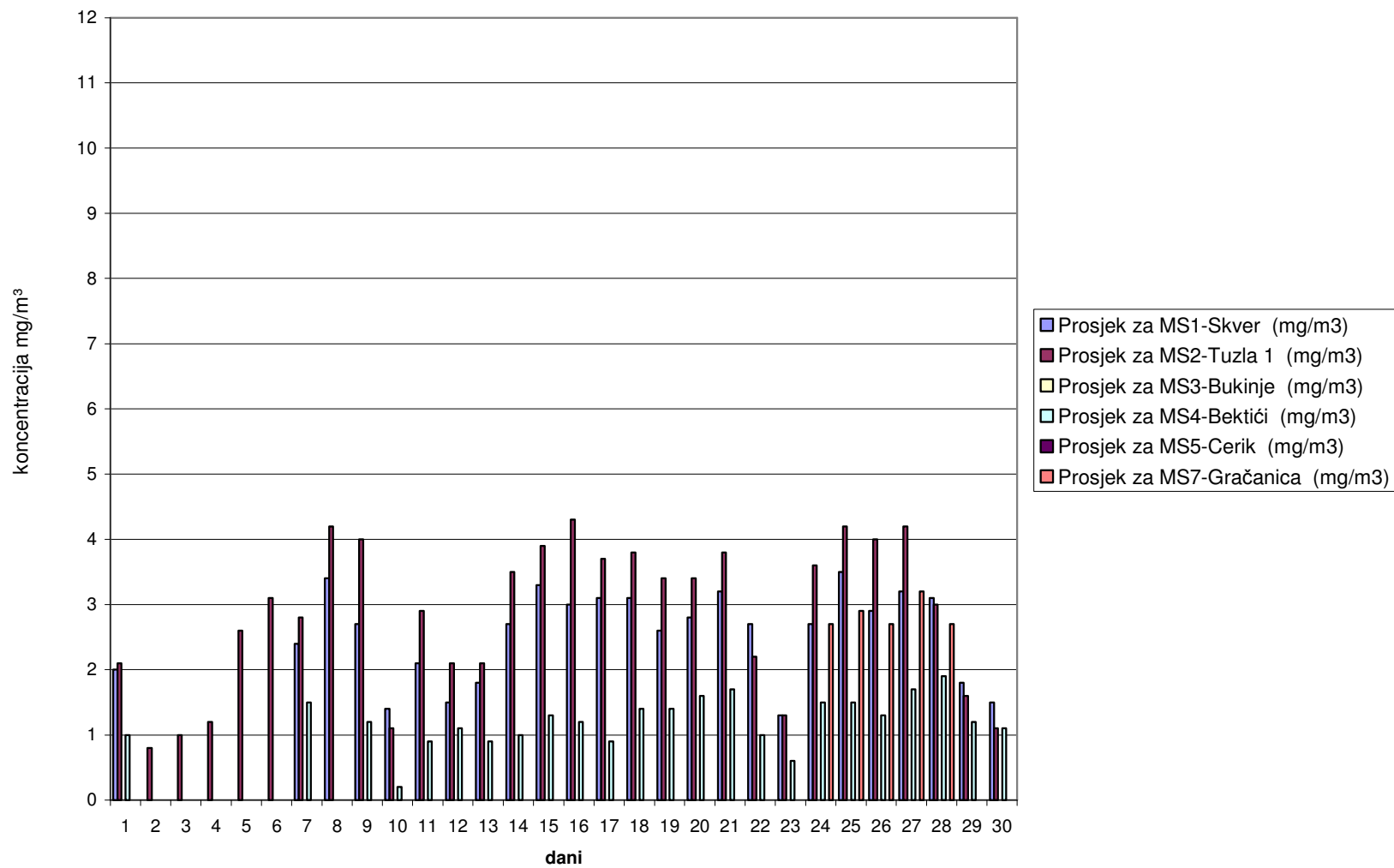
Slika 3. Grafički prikaz prosječnih dnevnih vrijednosti ugljenmonoksida (CO) za mjesec novembar/studeni 2006. godine
