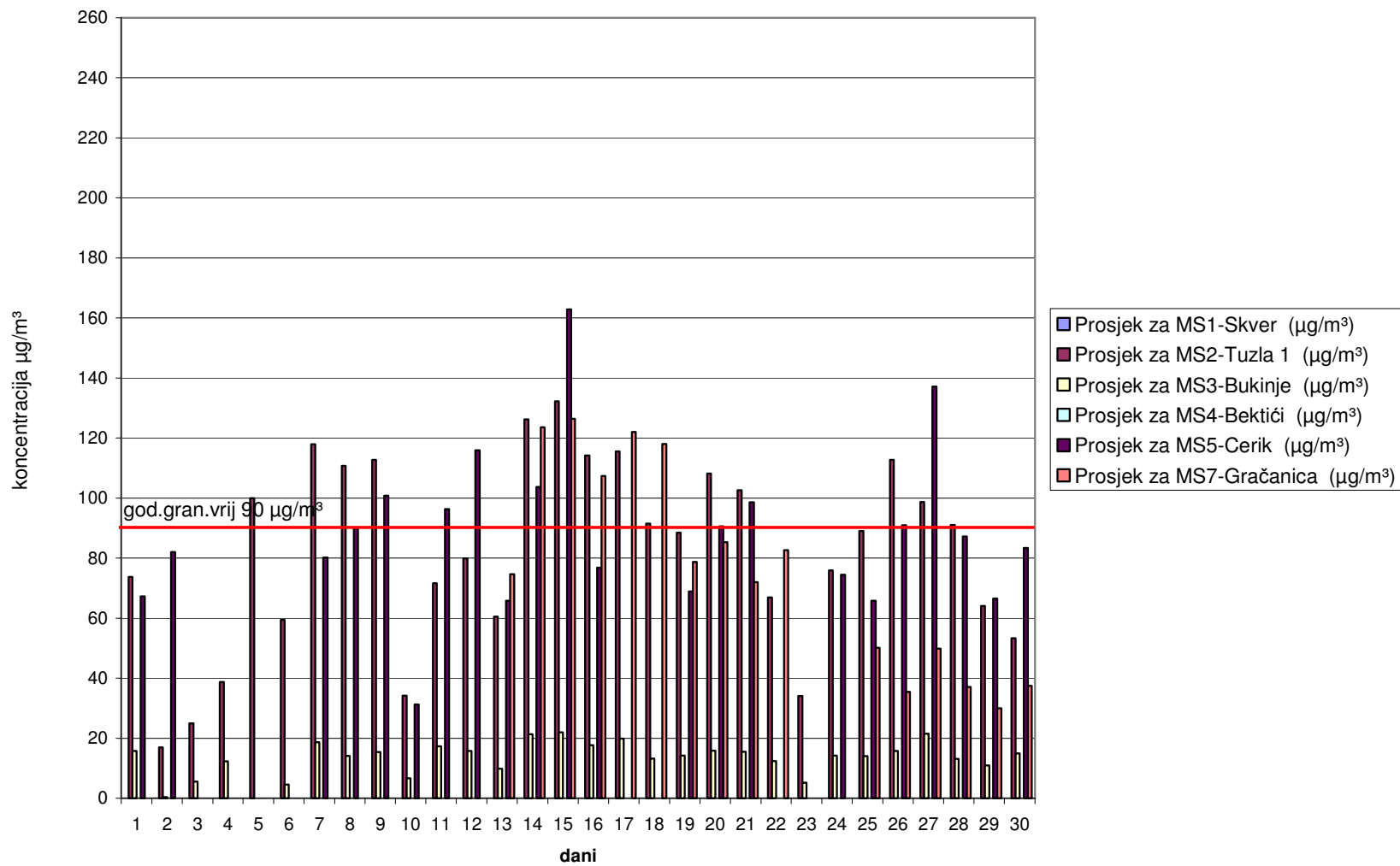
Slika 1. Grafički prikaz prosječnih dnevnih vrijednosti sumpordioksida (SO 2 ) za mjesec novembar/studeni 2006. godine
