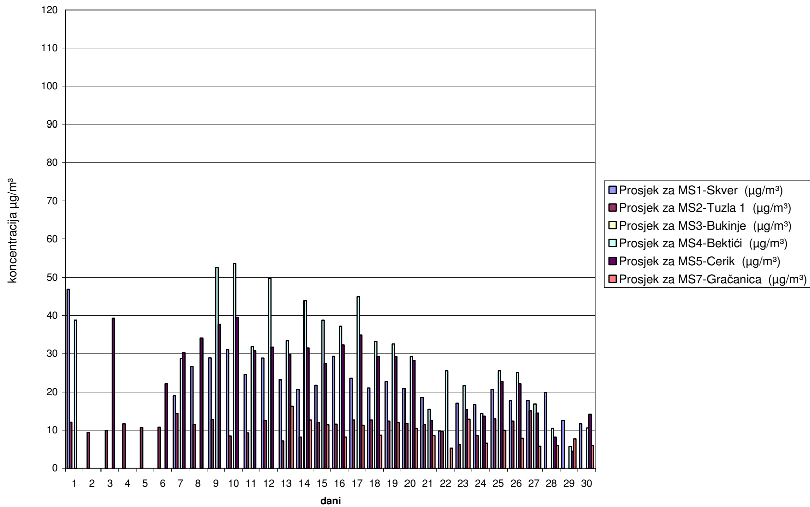
Slika 4. Grafički prikaz prosječnih dnevnih vrijednosti ozona ( \text{O}_3 ) za mjesec novembar/studenj 2006. godine
