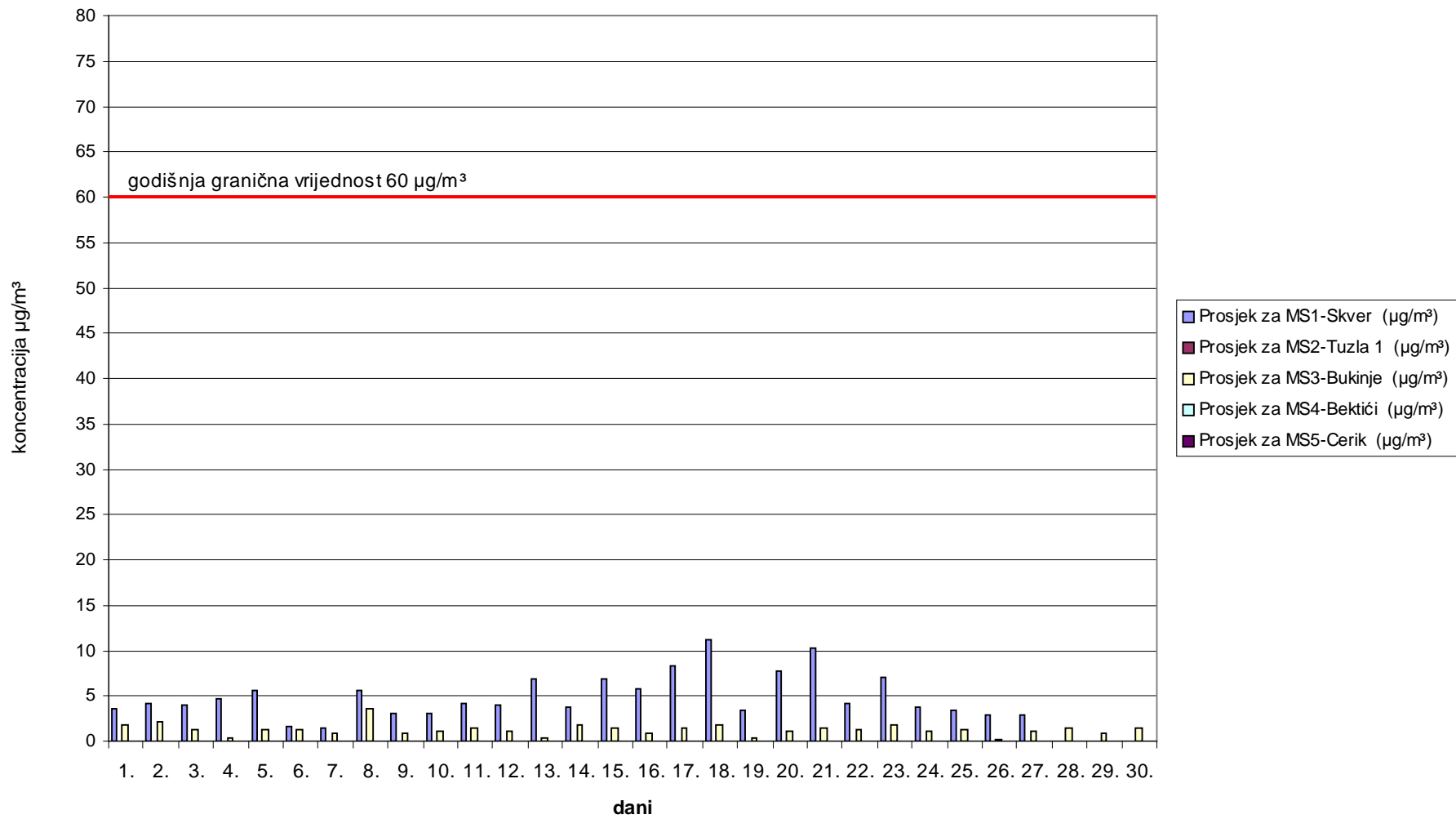
Slika 2. Grafički prikaz prosječnih dnevnih vrijednosti azotdioksida ( \text{NO}_2 ) za mjesec april 2008. godine
