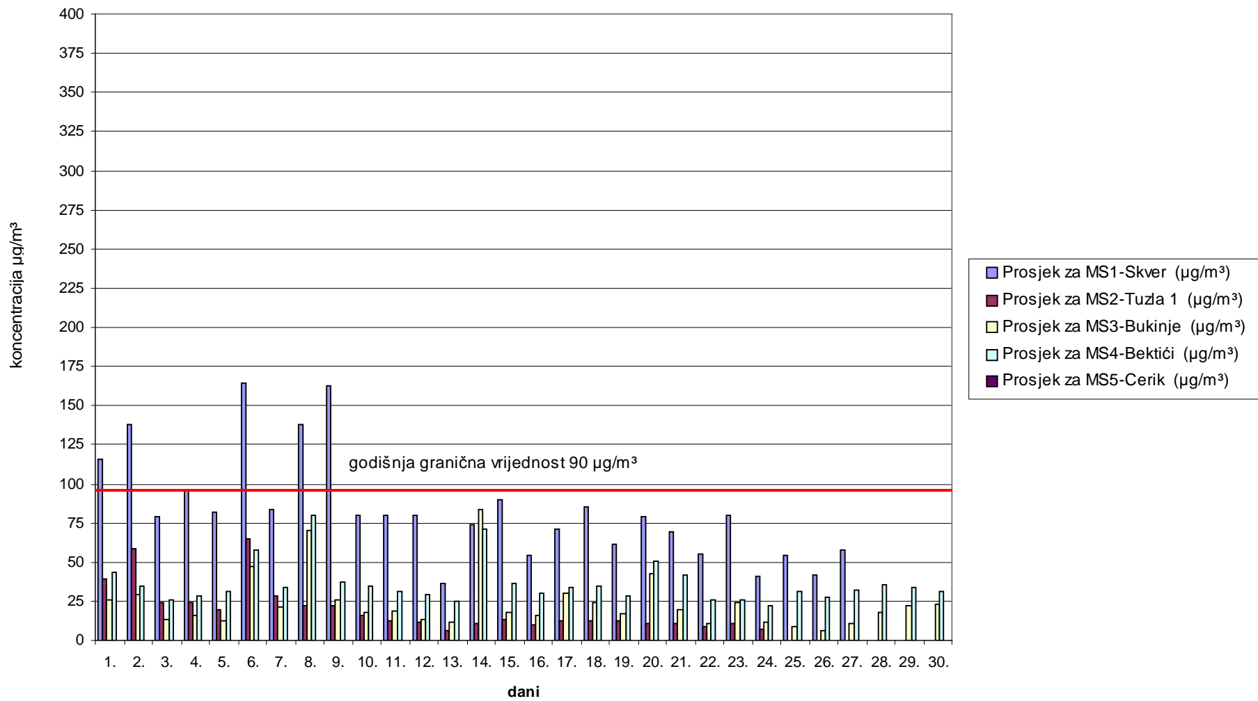
Slika 1. Grafički prikaz prosječnih dnevnih vrijednosti sumpordioksida (SO 2 ) za mjesec april 2008. godine
