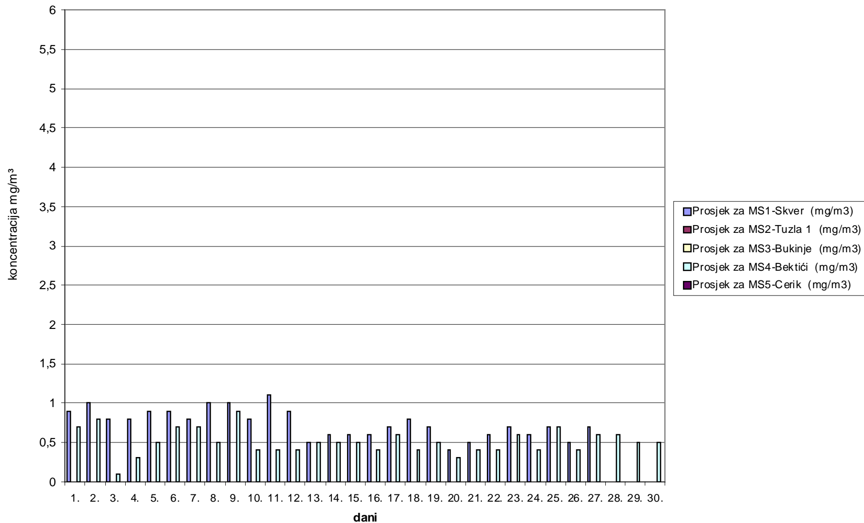
Slika 3. Grafički prikaz prosječnih dnevni vrijednosti ugljenmonoksida (CO) za mjesec april 2008. godine
