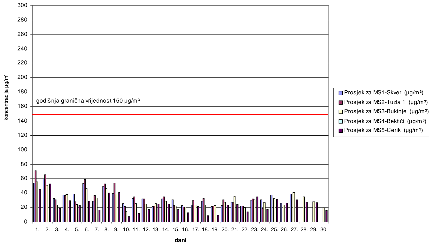
Slika 5. Grafički prikaz prosječnih dnevnih vrijednosti lebdećih čestica ( \text{PM}_{2,5} ) za mjesec april/travanj 2008. godine
