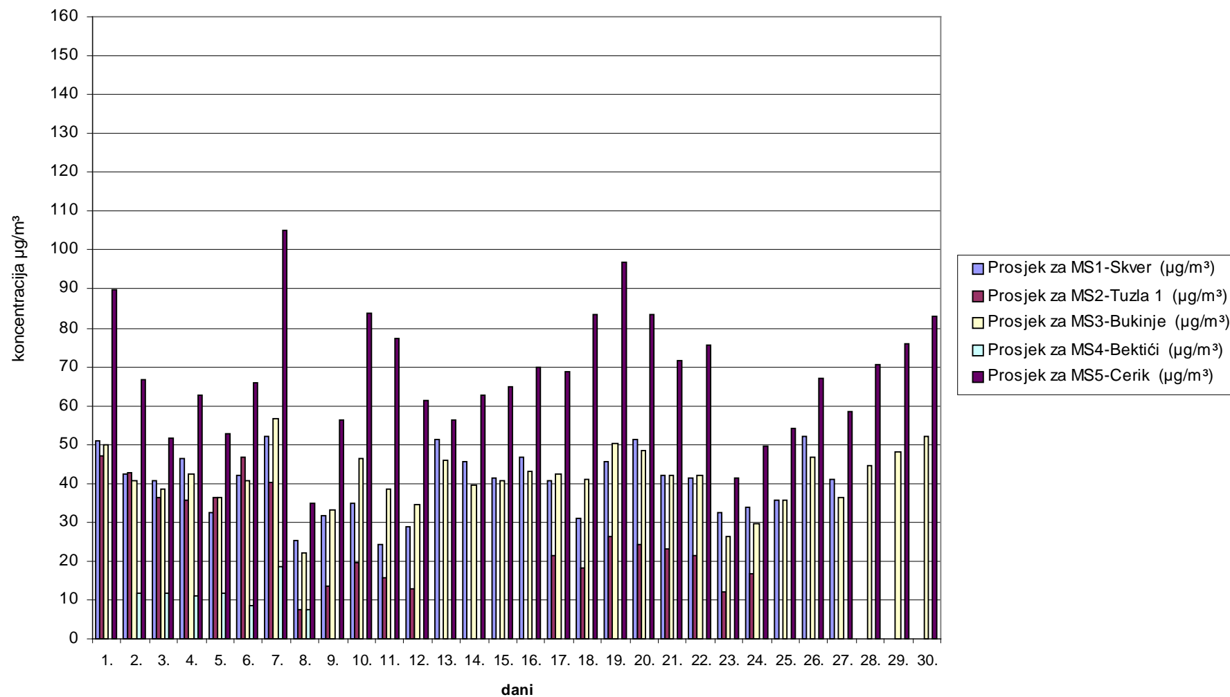
Slika 4. Grafički prikaz prosječnih dnevnih vrijednosti ozona ( \text{O}_3 ) za mjesec april 2008. godine
