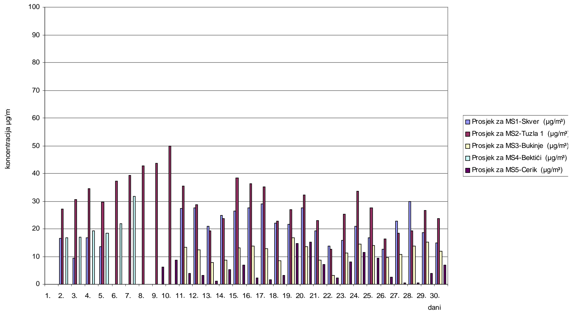
Slika 2. Grafički prikaz prosječnih dnevni vrijednosti azotdioksida (NO 2 ) za mjesec april/travanj 2009. godine
