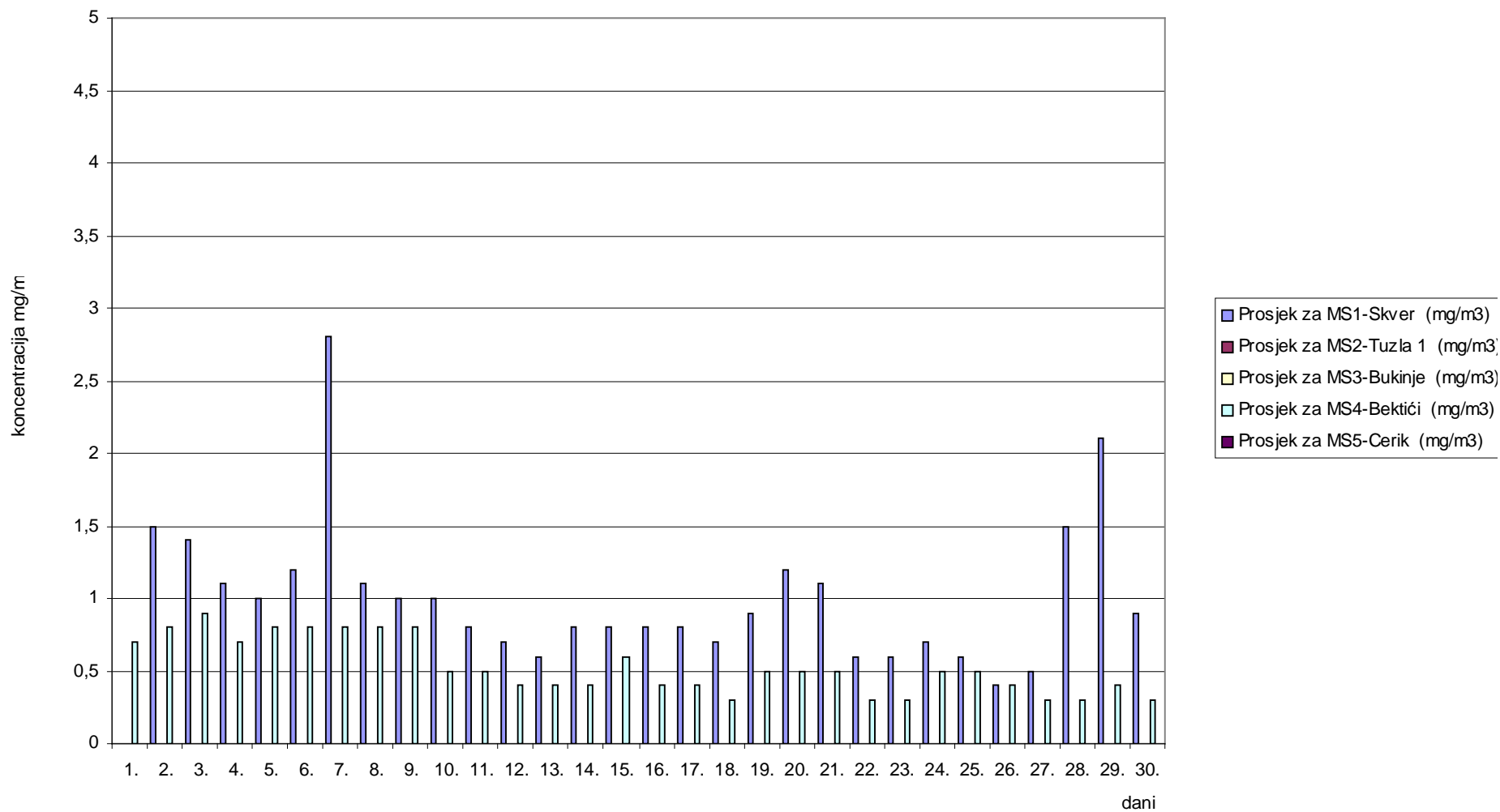
Slika 3. Grafički prikaz prosječnih dnevnih vrijednosti ugljenmonoksida (CO) za mjesec april/travanj 2009. godine
