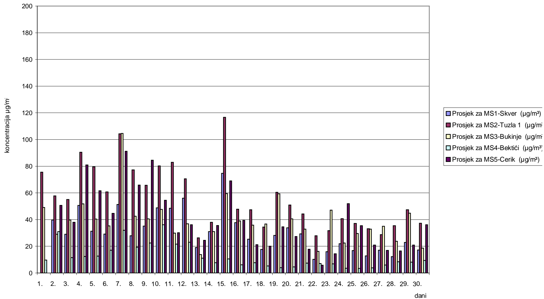
Slika 1. Grafički prikaz prosječnih dnevnih vrijednosti sumpordioksida ( \text{SO}_2 ) za mjesec april/travanj 2009. godine
