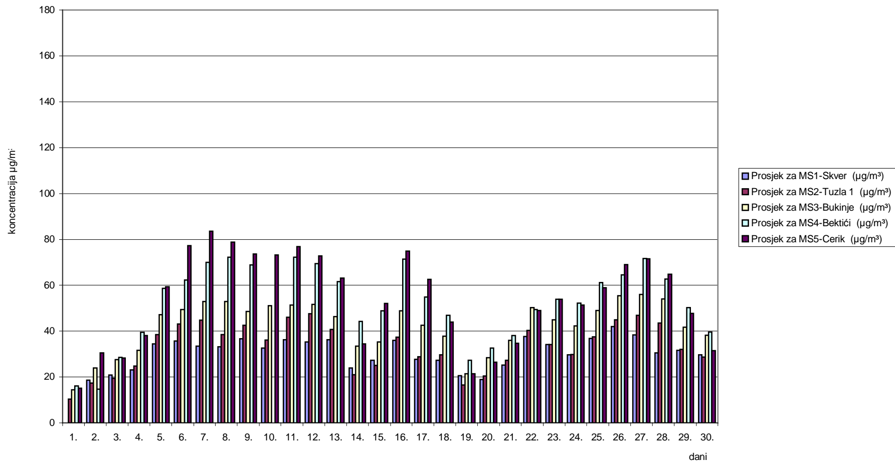
Slika 4. Grafički prikaz prosječnih dnevni vrijednosti ozona (O 3 ) za mjesec april/travanj 2009. godine
