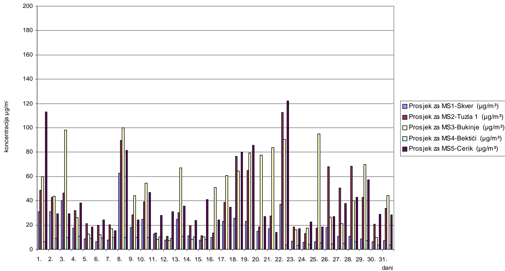
Slika 1. Grafički prikaz prosječnih dnevnih vrijednosti sumpordioksida (SO 2 ) za mjesec avgust/kolovoz 2009. godine
