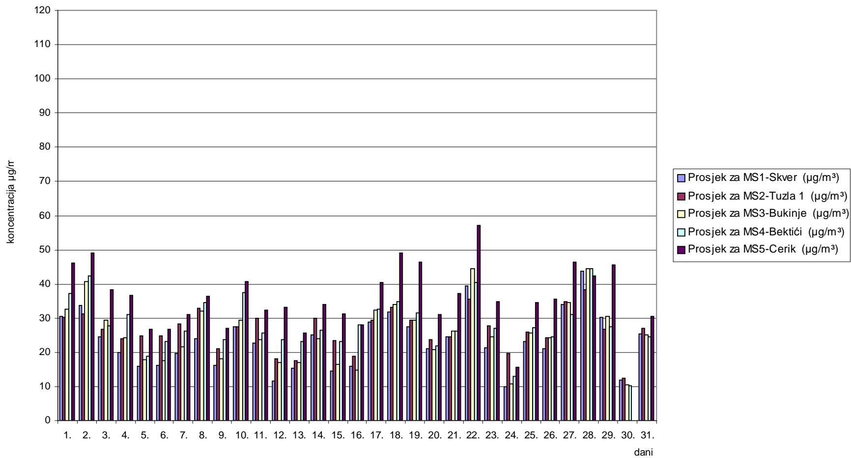
Slika 5. Grafički prikaz prosječnih dnevni vrijednosti lebdećih čestica (PM 2,5 ) za mjesec avgust/kolovoz 2009. godine
