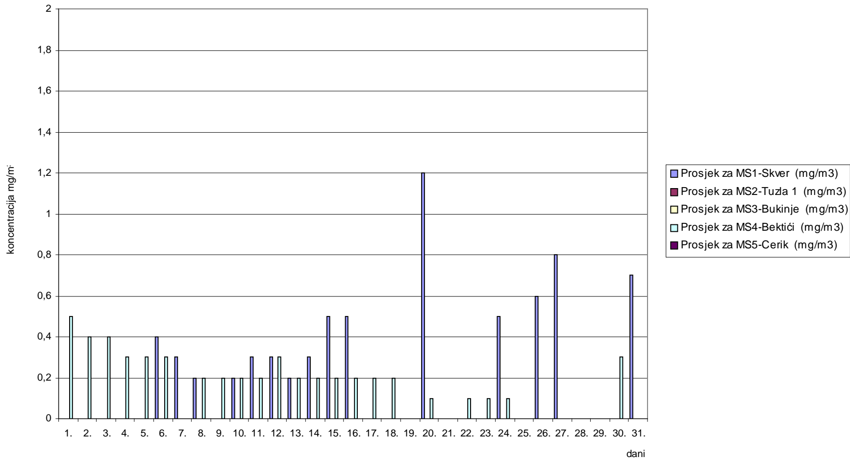
Slika 3. Grafički prikaz prosječnih dnevnih vrijednosti ugljenmonoksida (CO) za mjesec avgust/kolovoz 2009. godine
