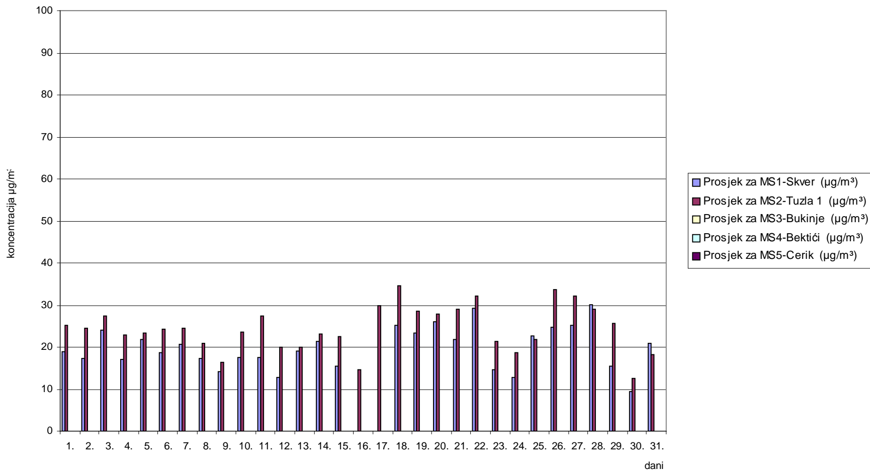
Slika 2. Grafički prikaz prosječnih dnevni vrijednosti azotdioksida (NO 2 ) za mjesec avgust/kolovoz 2009. godine
