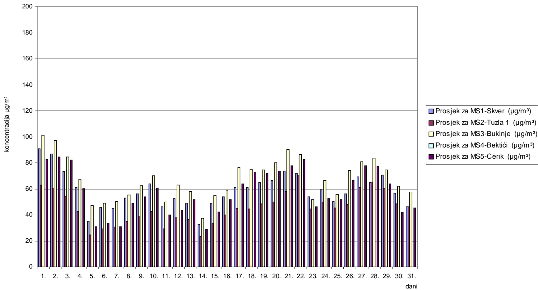
Slika 4. Grafički prikaz prosječnih dnevnih vrijednosti ozona (O 3 ) za mjesec avgust/kolovoz 2009. godine
