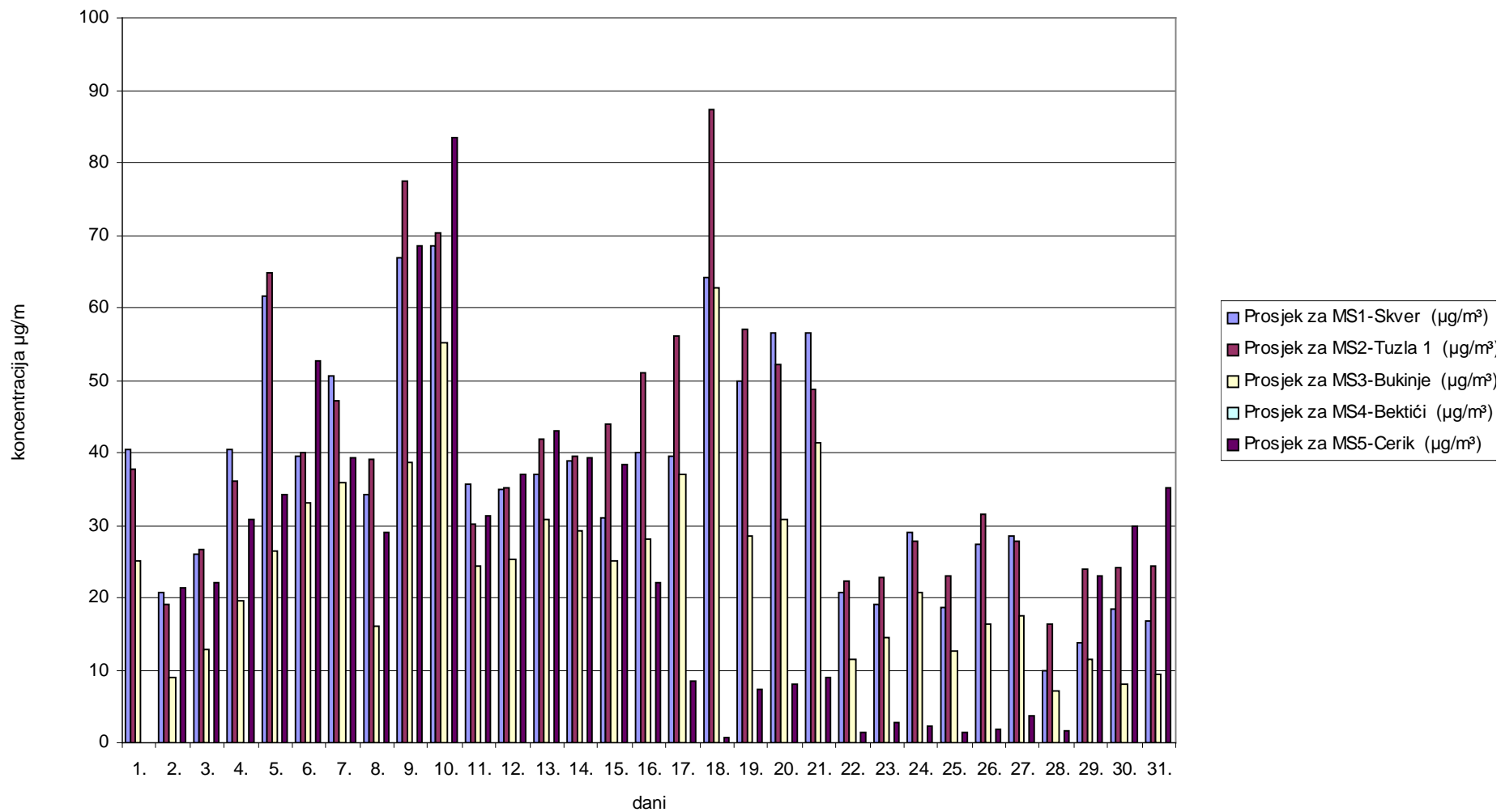
Slika 2. Grafički prikaz prosječnih dnevnih vrijednosti azotdioksida (NO 2 ) za mjesec januar/siječanj 2009. godine
