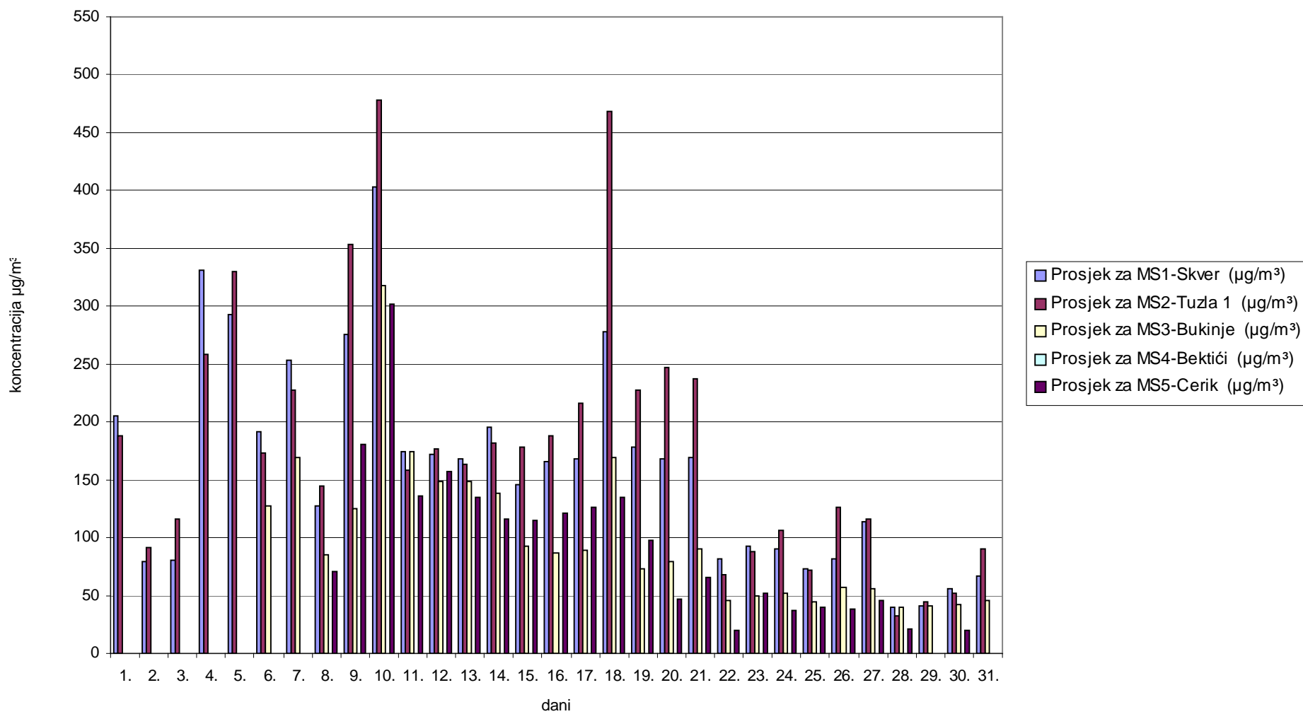
Slika 1. Grafički prikaz prosječnih dnevnih vrijednosti sumpordioksida (SO 2 ) za mjesec januar/siječanj 2009. godine
