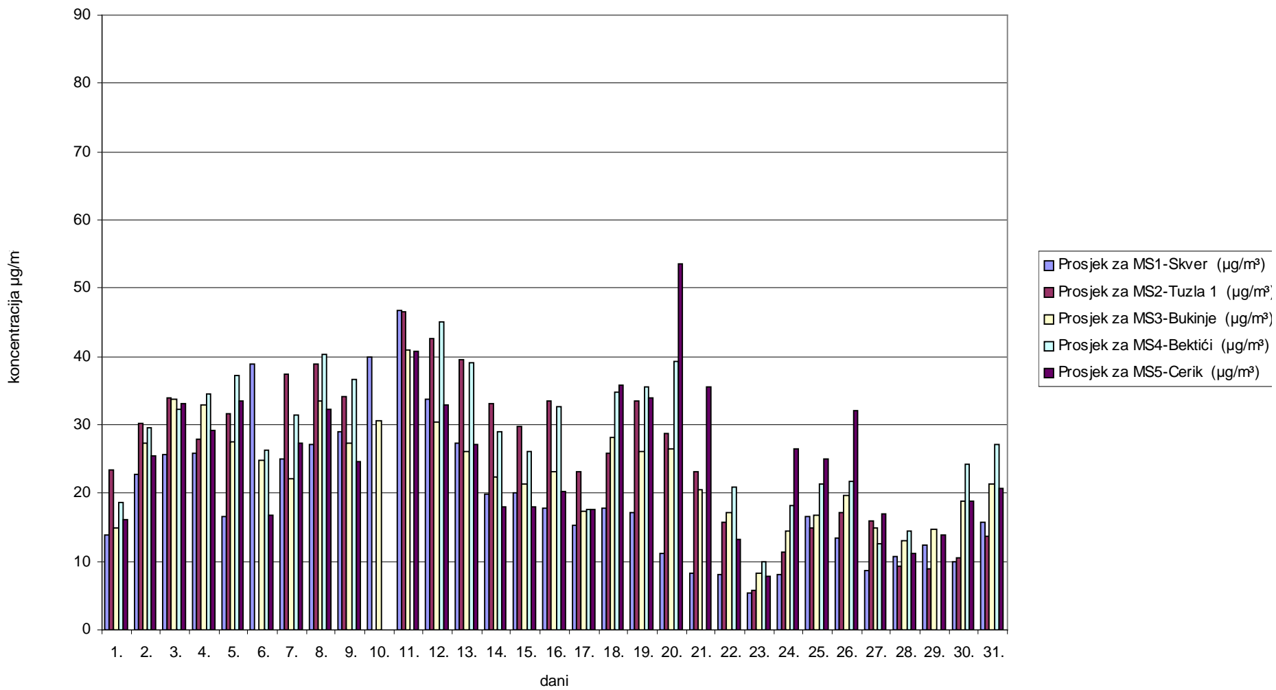
Slika 4. Grafički prikaz prosječnih dnevnih vrijednosti ozona ( O_3 ) za mjesec januar/siječanj 2009. godine
