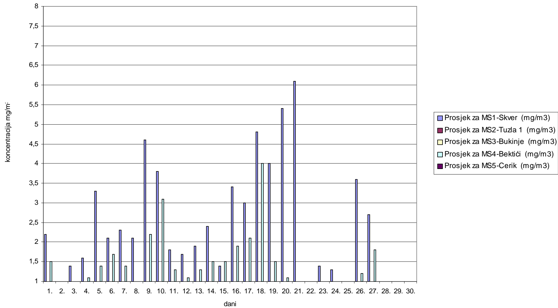
Slika 3. Grafički prikaz prosječnih dnevnih vrijednosti ugljenmonoksida (CO) za mjesec januar/siječanj 2009. godine
