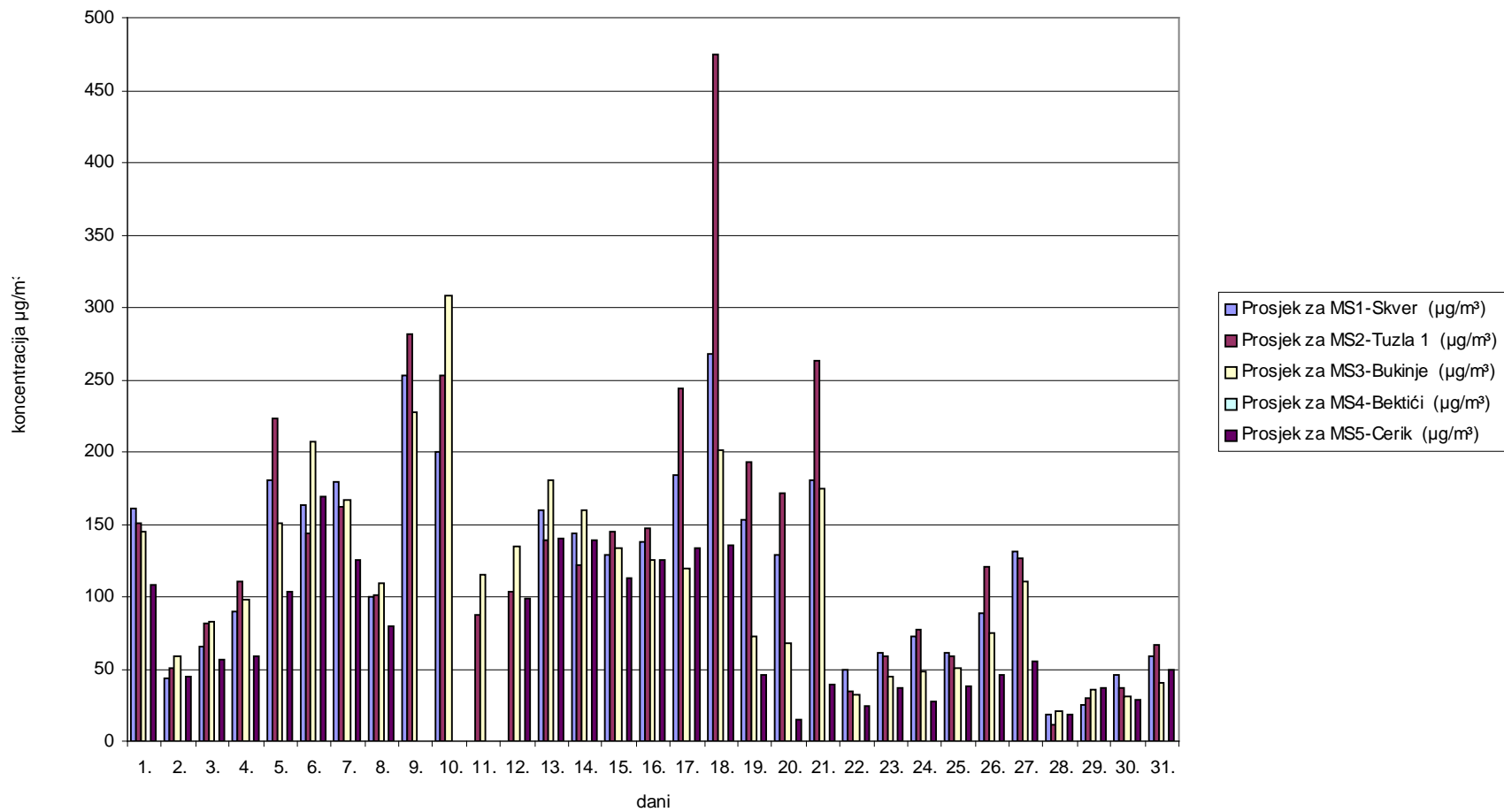
Slika 5. Grafički prikaz prosječnih dnevnih vrijednosti lebdećih čestica (PM 2,5 ) za mjesec januar/siječanj 2009. godine
