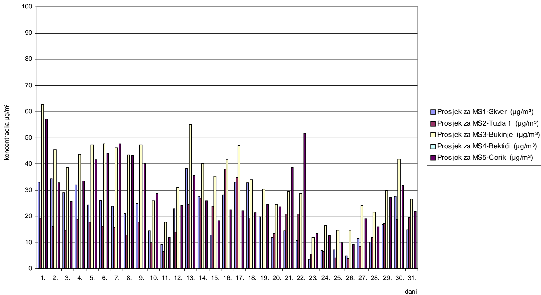
Slika 4. Grafički prikaz prosječnih dnevni vrijednosti ozona (O 3 ) za mjesec oktobar/listopad 2009. godine
