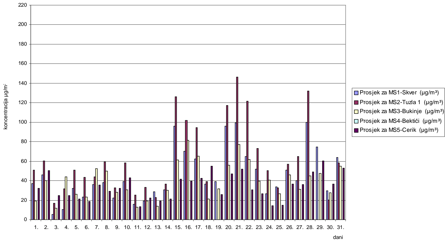
Slika 1. Grafički prikaz prosječnih dnevni vrijednosti sumpordioksida (SO 2 ) za mjesec oktobar/listopad 2009. godine
