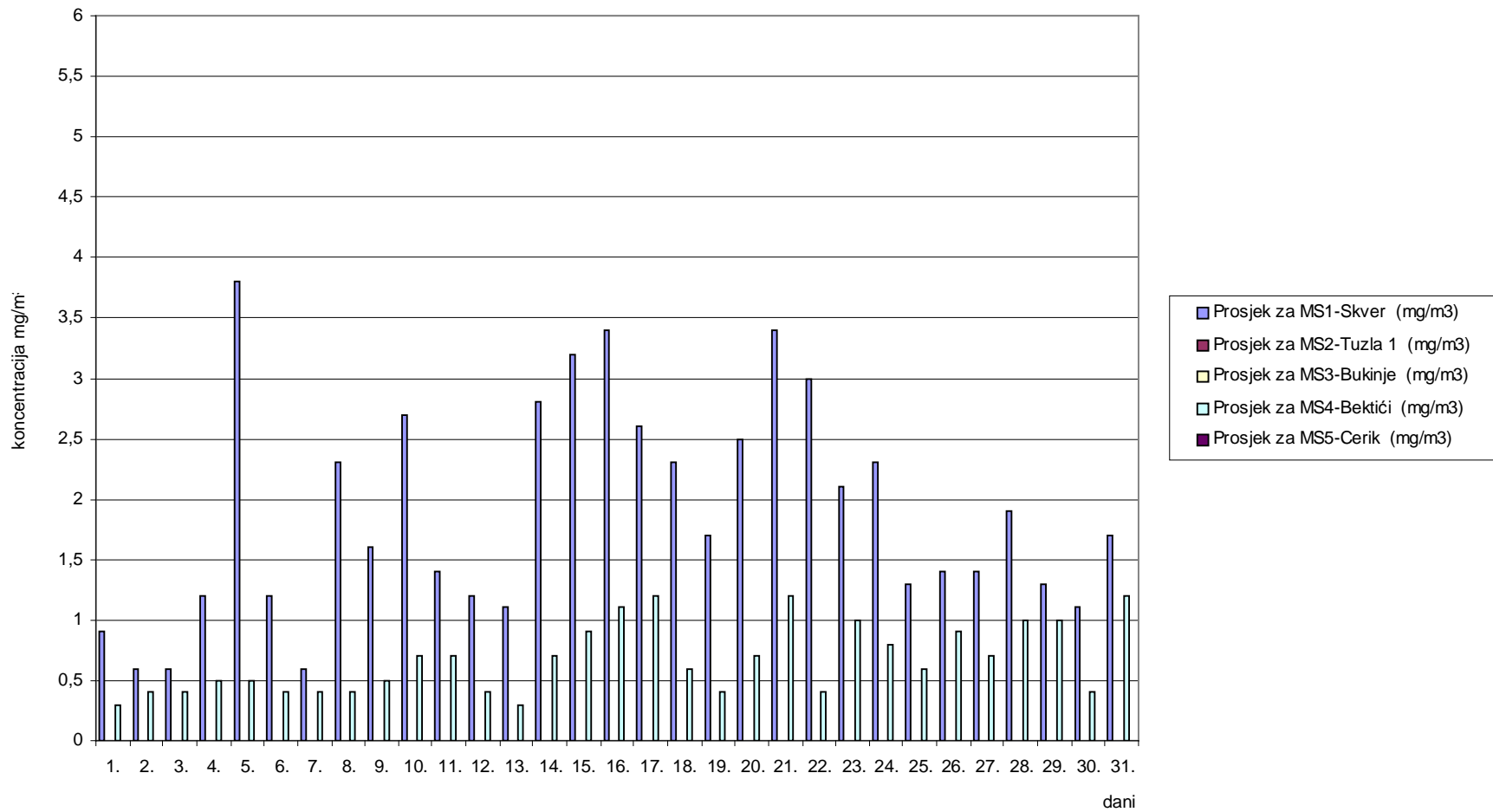
Slika 3. Grafički prikaz prosječnih dnevni vrijednosti ugljenmonoksida (CO) za mjesec oktobar/listopad 2009. godine
