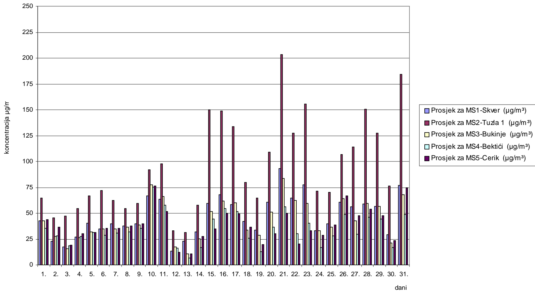
Slika 5. Grafički prikaz prosječnih dnevnih vrijednosti lebdećih čestica (PM 2,5 ) za mjesec oktobar/listopad 2009. godine
