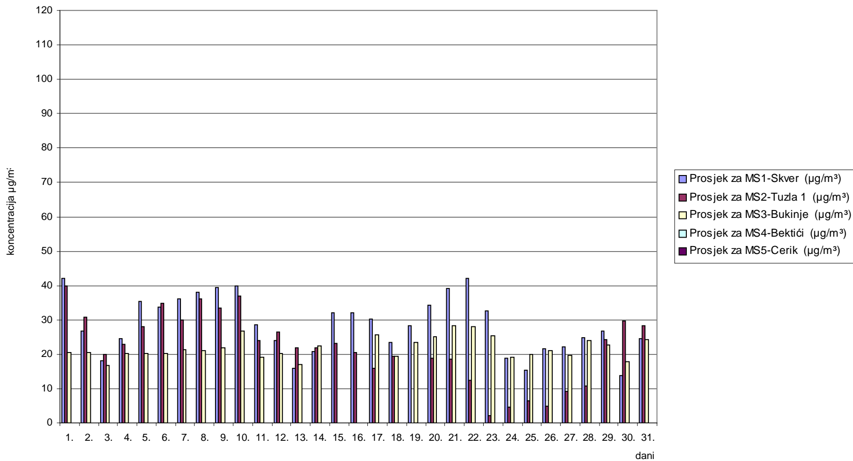
Slika 2. Grafički prikaz prosječnih dnevnih vrijednosti azotdioksida ( \text{NO}_2 ) za mjesec oktobar/listopad 2009. godine
