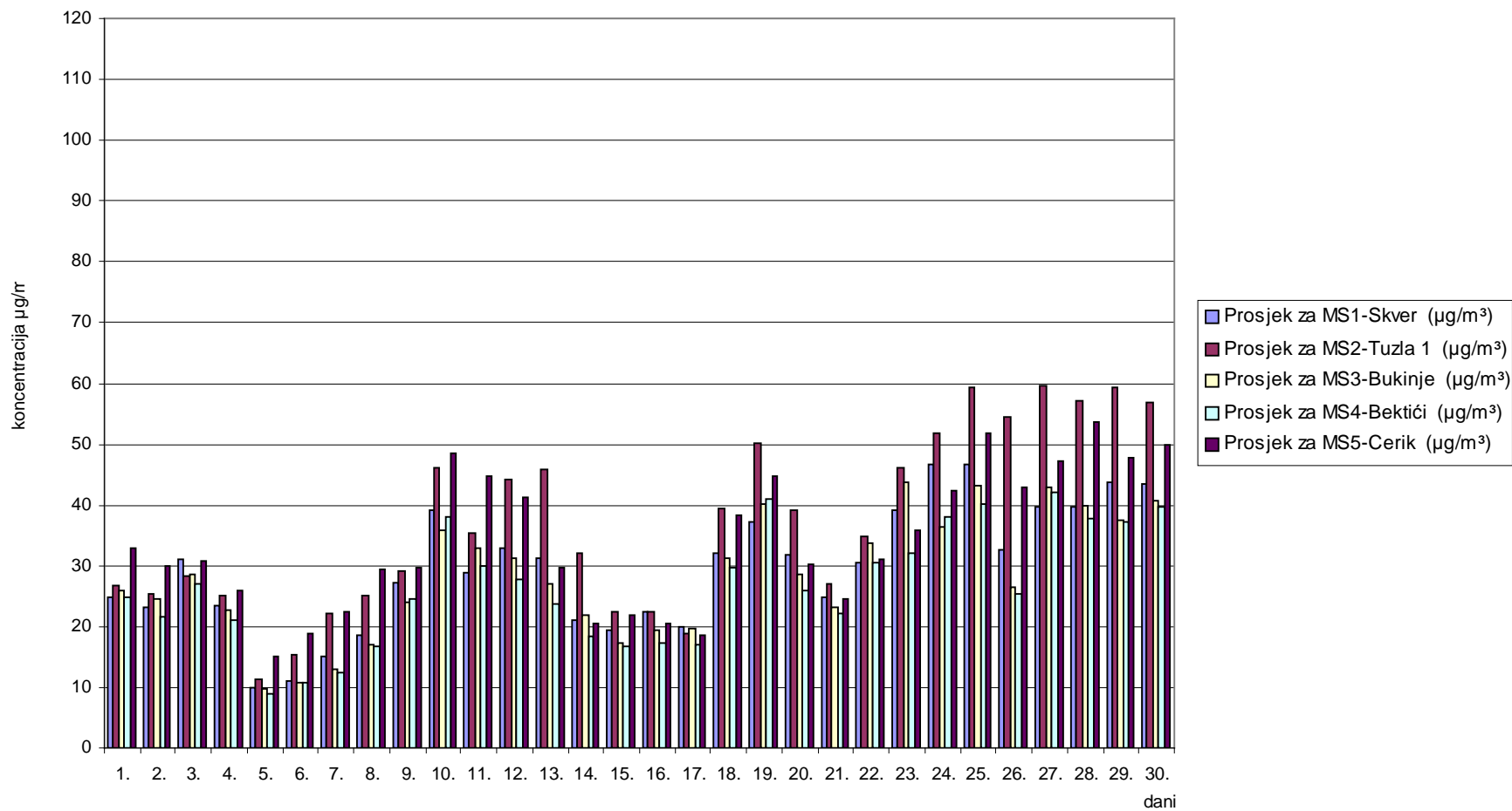
Slika 5. Grafički prikaz prosječnih dnevni vrijednosti lebdećih čestica (PM 2,5 ) za mjesec septembar/rujan 2009. godine
