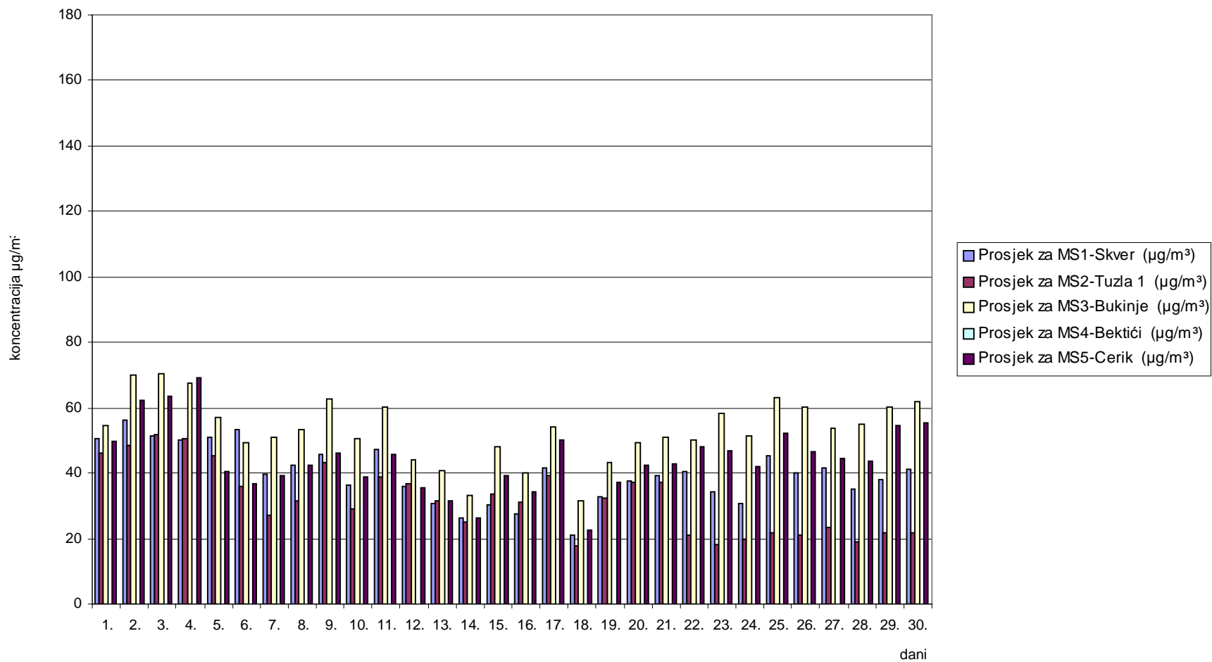
Slika 4. Grafički prikaz prosječnih dnevni vrijednosti ozona (O 3 ) za mjesec septembar/rujan 2009. godine
