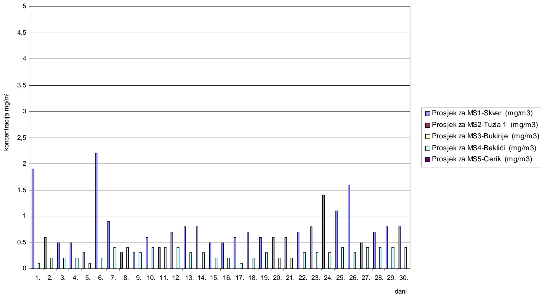
Slika 3. Grafički prikaz prosječnih dnevnih vrijednosti ugljenmonoksida (CO) za mjesec septembar/rujan 2009. godine
