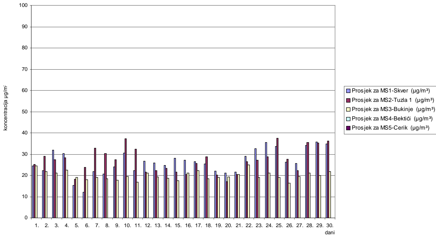
Slika 2. Grafički prikaz prosječnih dnevni vrijednosti azotdioksida ( \text{NO}_2 ) za mjesec septembar/rujan 2009. godine
