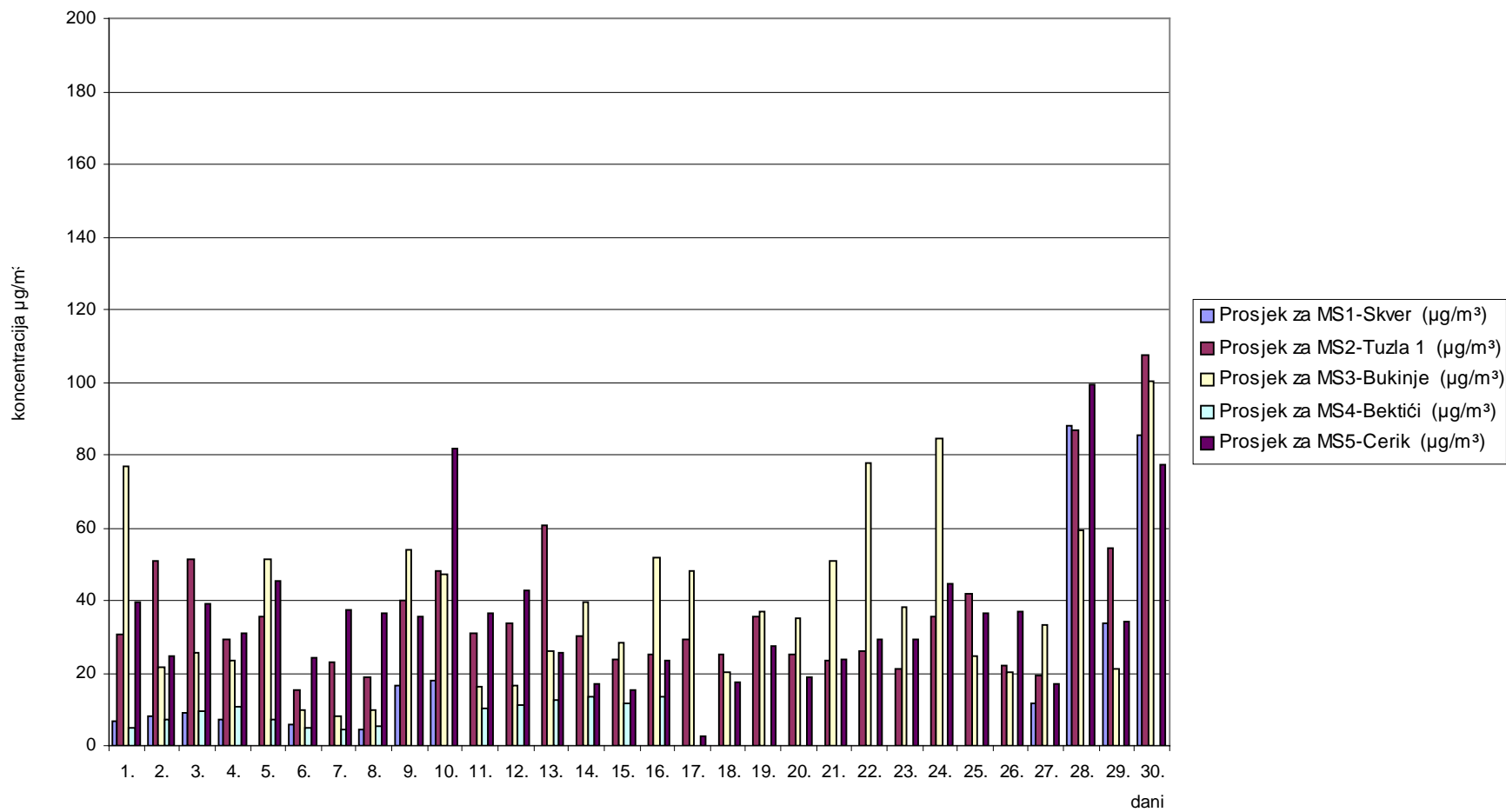
Slika 1. Grafički prikaz prosječnih dnevni vrijednosti sumpordioksida (SO 2 ) za mjesec septembar/rujan 2009. godine
