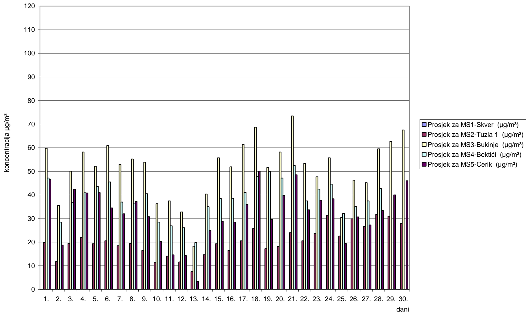
Slika 4. Grafički prikaz prosječnih dnevnih vrijednosti ozona (O 3 ) za mjesec april/travanj 2010. godine
