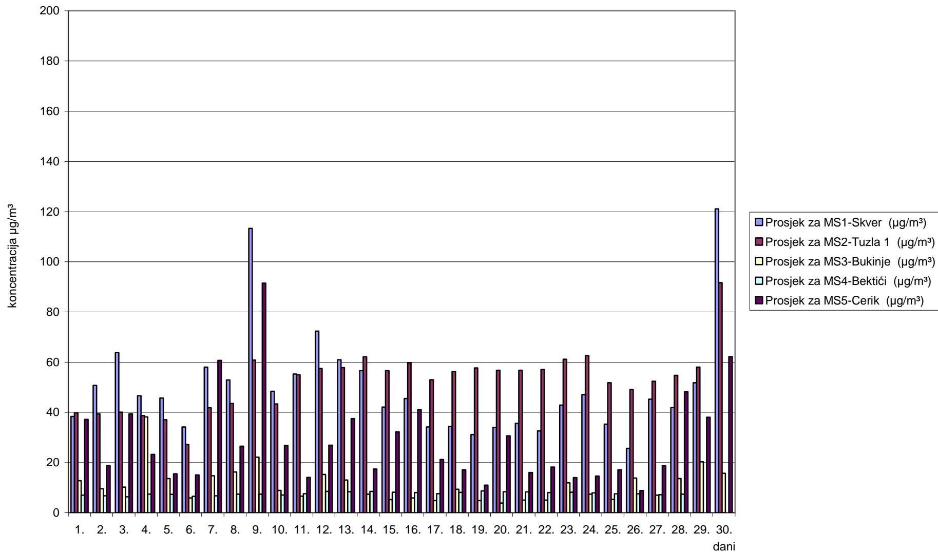
Slika 1. Grafički prikaz prosječnih dnevnih vrijednosti sumpordioksida (SO 2 ) za mjesec april/travanj 2010. godine
