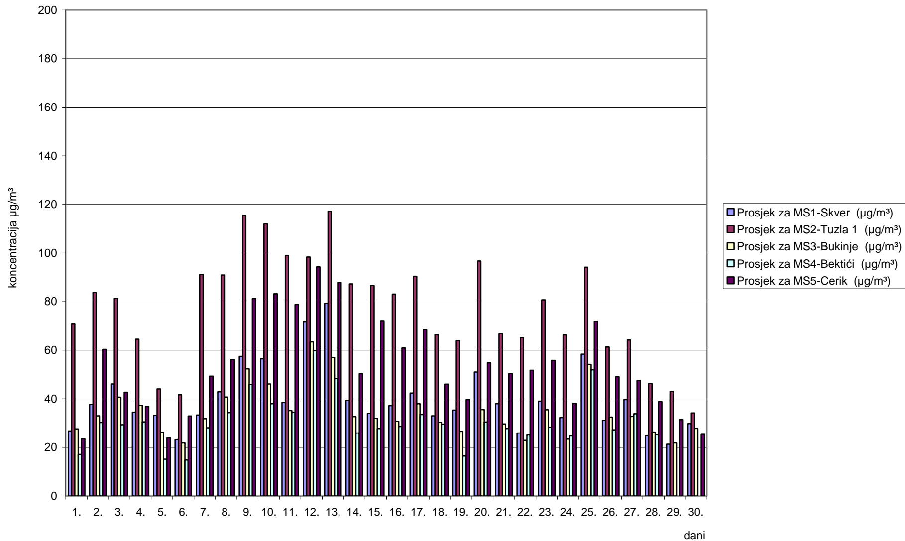
Slika 5. Grafički prikaz prosječnih dnevnih vrijednosti lebdećih čestica (PM 2.5 ) za mjesec april/travanj 2010. godine
