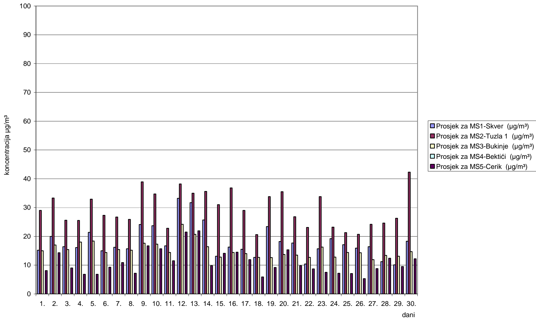
Slika 2. Grafički prikaz prosječnih dnevnih vrijednosti azotdioksida (NO 2 ) za mjesec april/travanj 2010. godine
