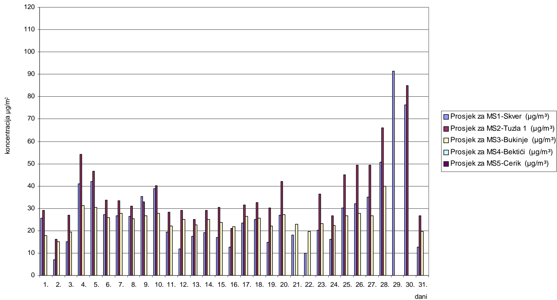
Slika 2. Grafički prikaz prosječnih dnevnih vrijednosti azotdioksida (NO 2 ) za mjesec januar/siječanj 2010. godine
