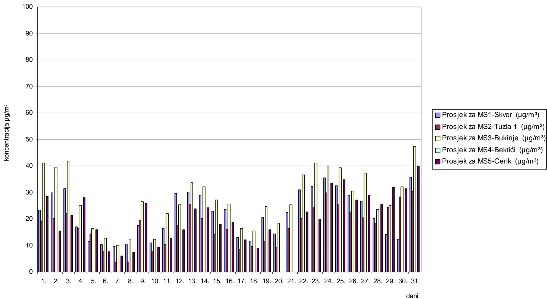
Slika 4. Grafički prikaz prosječnih dnevnih vrijednosti ozona (O 3 ) za mjesec januar/siječanj 2010. godine
