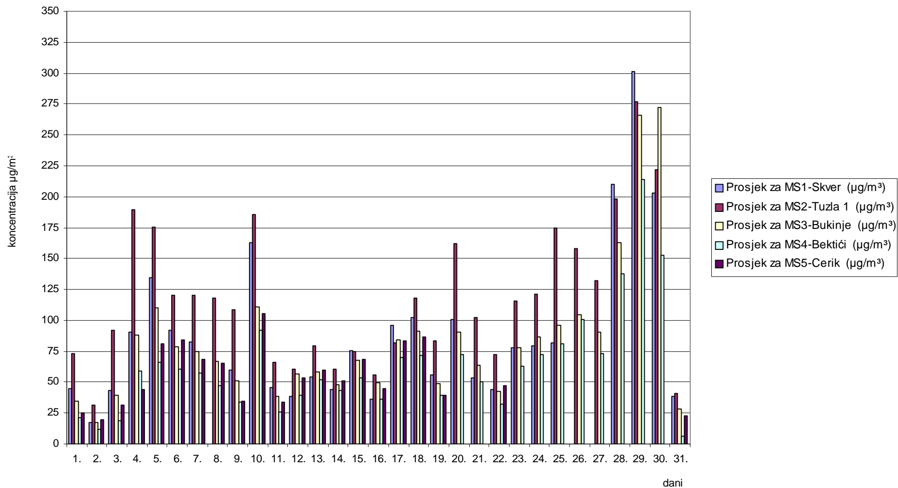
Slika 5. Grafički prikaz prosječnih dnevnih vrijednosti lebdećih čestica (PM 2,5 ) za mjesec januar/siječanj 2010. godine
