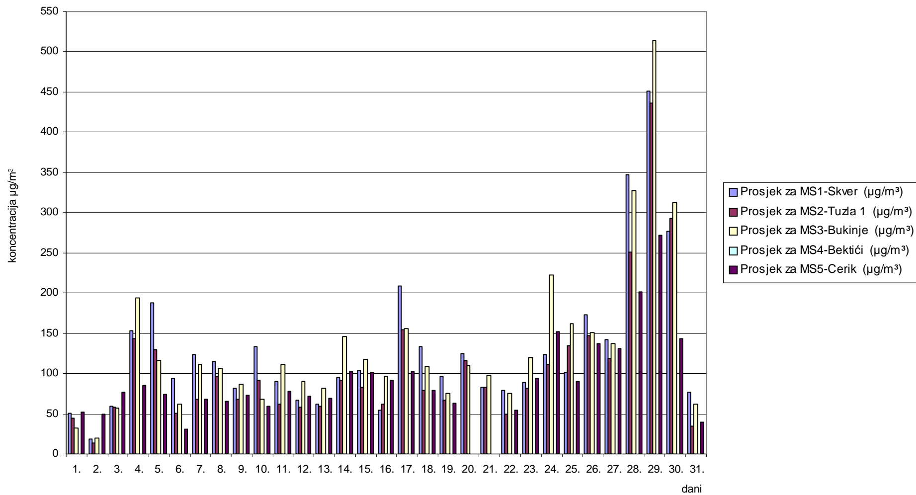
Slika 1. Grafički prikaz prosječnih dnevnih vrijednosti sumpordioksida (SO 2 ) za mjesec januar/siječanj 2010. godine
