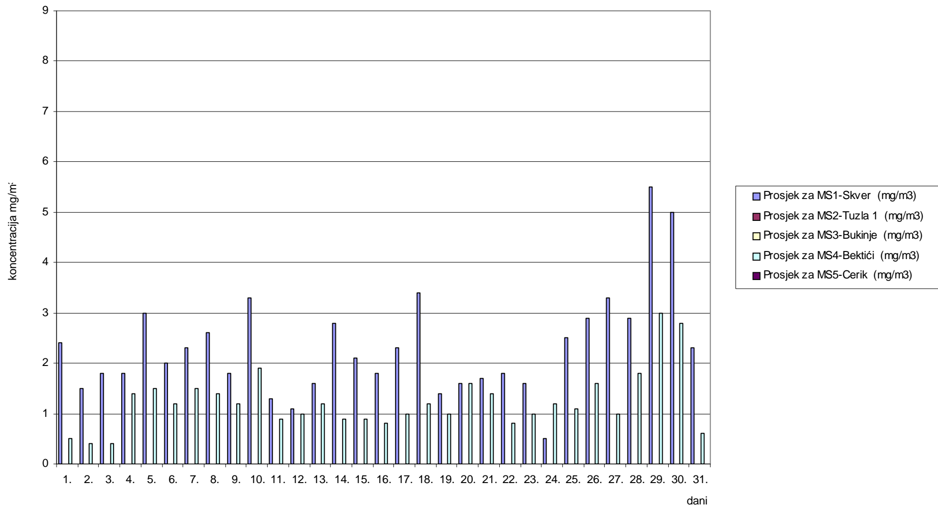
Slika 3. Grafički prikaz prosječnih dnevnih vrijednosti ugljenmonoksida (CO) za mjesec januar/siječanj 2010. godine
