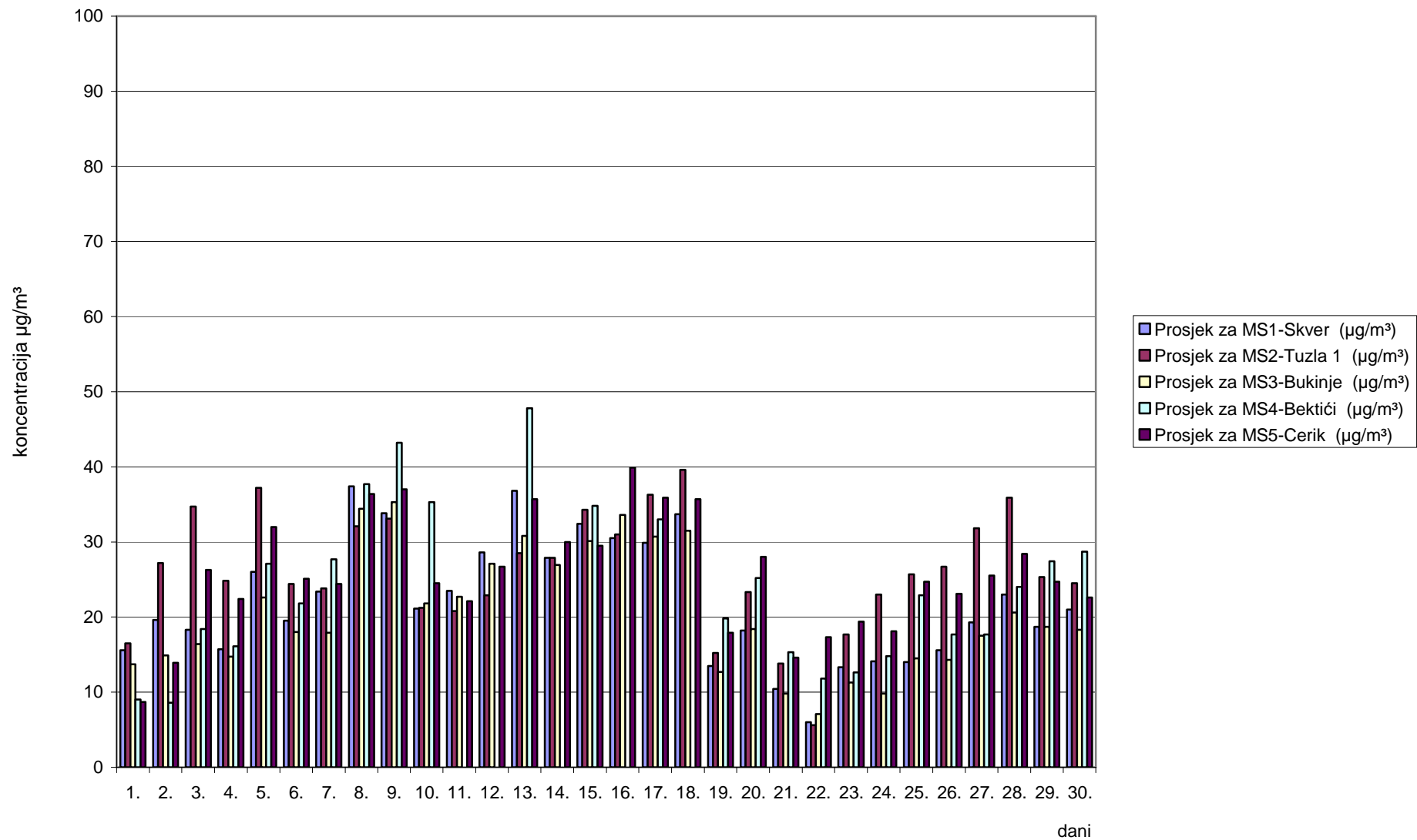
Slika 5. Grafički prikaz prosječnih dnevnih vrijednosti lebdećih čestica (PM 2.5 ) za mjesec juni/lipanj 2010. godine
