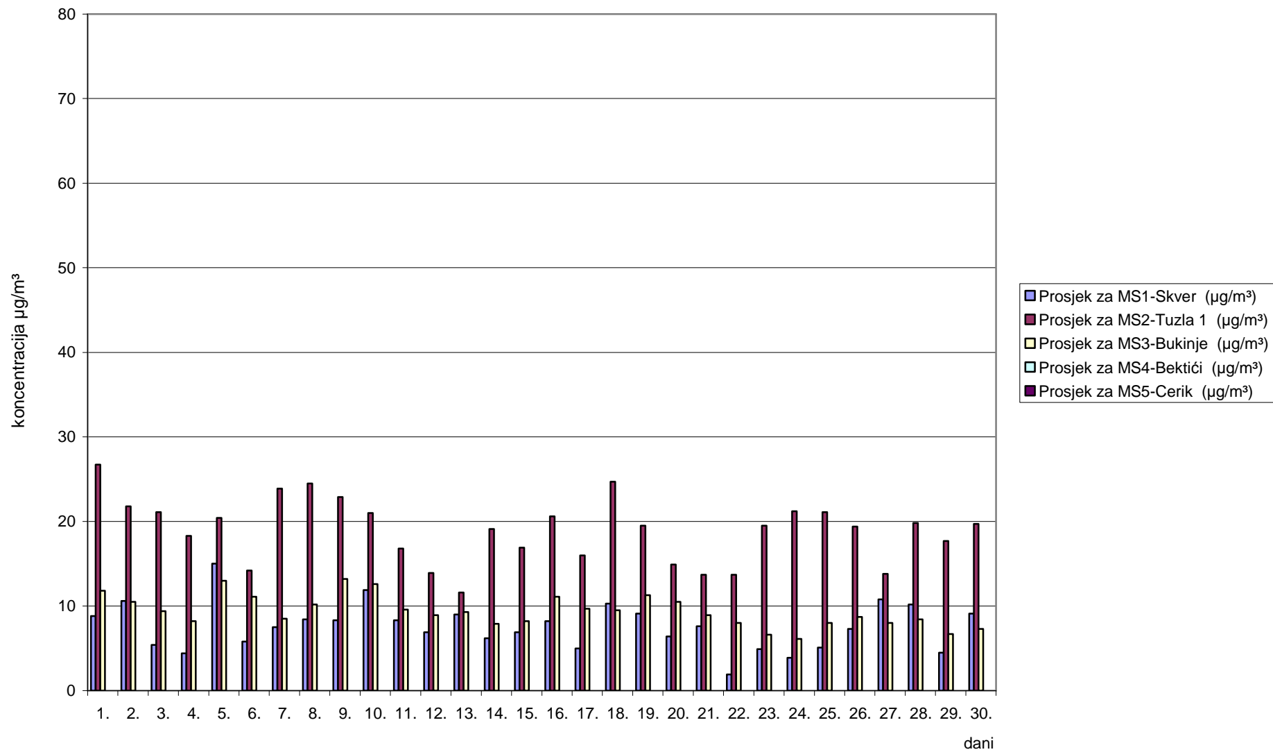
Slika 2. Grafički prikaz prosječnih dnevnih vrijednosti azotdioksida ( \text{NO}_2 ) za mjesec juni/lipanj 2010. godine
