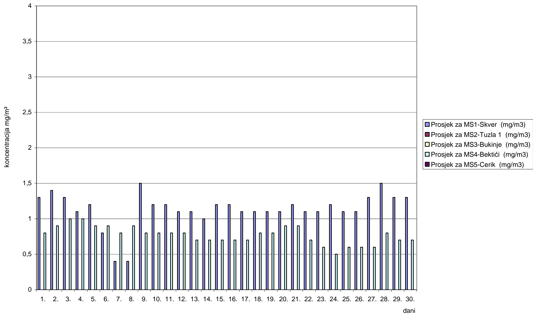
Slika 3. Grafički prikaz prosječnih dnevnih vrijednosti ugljenmonoksida (CO) za mjesec juni/lipanj 2010. godine
