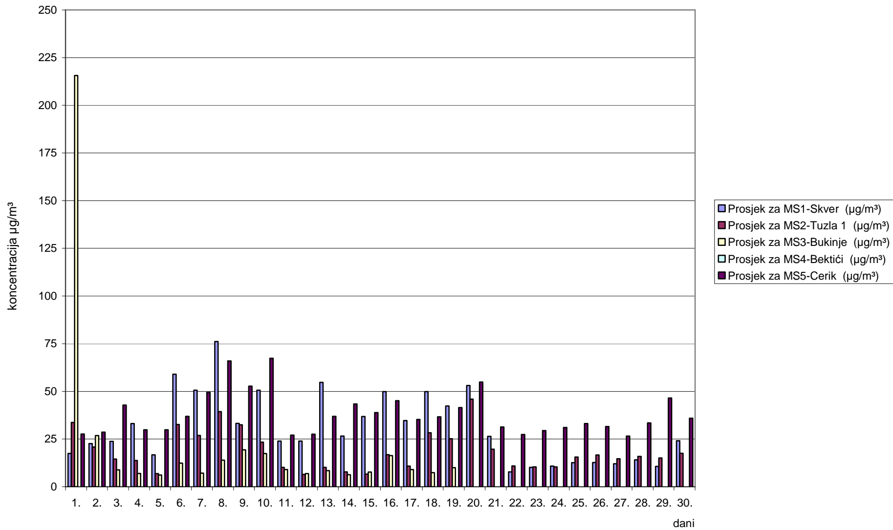
Slika 1. Grafički prikaz prosječnih dnevnih vrijednosti sumpordioksida ( \text{SO}_2 ) za mjesec juni/lipanj 2010. godine
