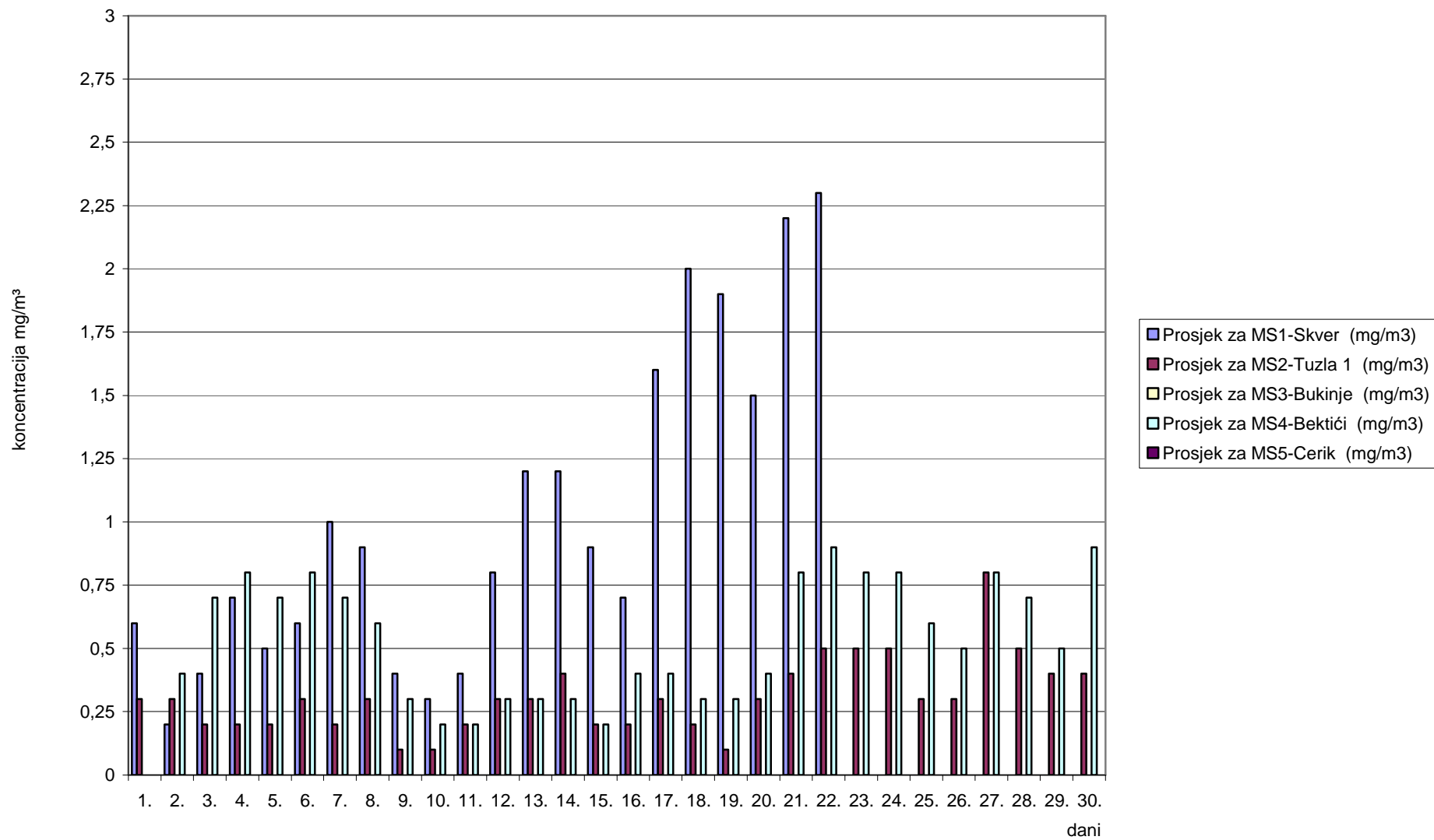
Slika 3. Grafički prikaz prosječnih dnevnih vrijednosti ugljenmonoksida (CO) za mjesec septembar/rujan 2010. godine
