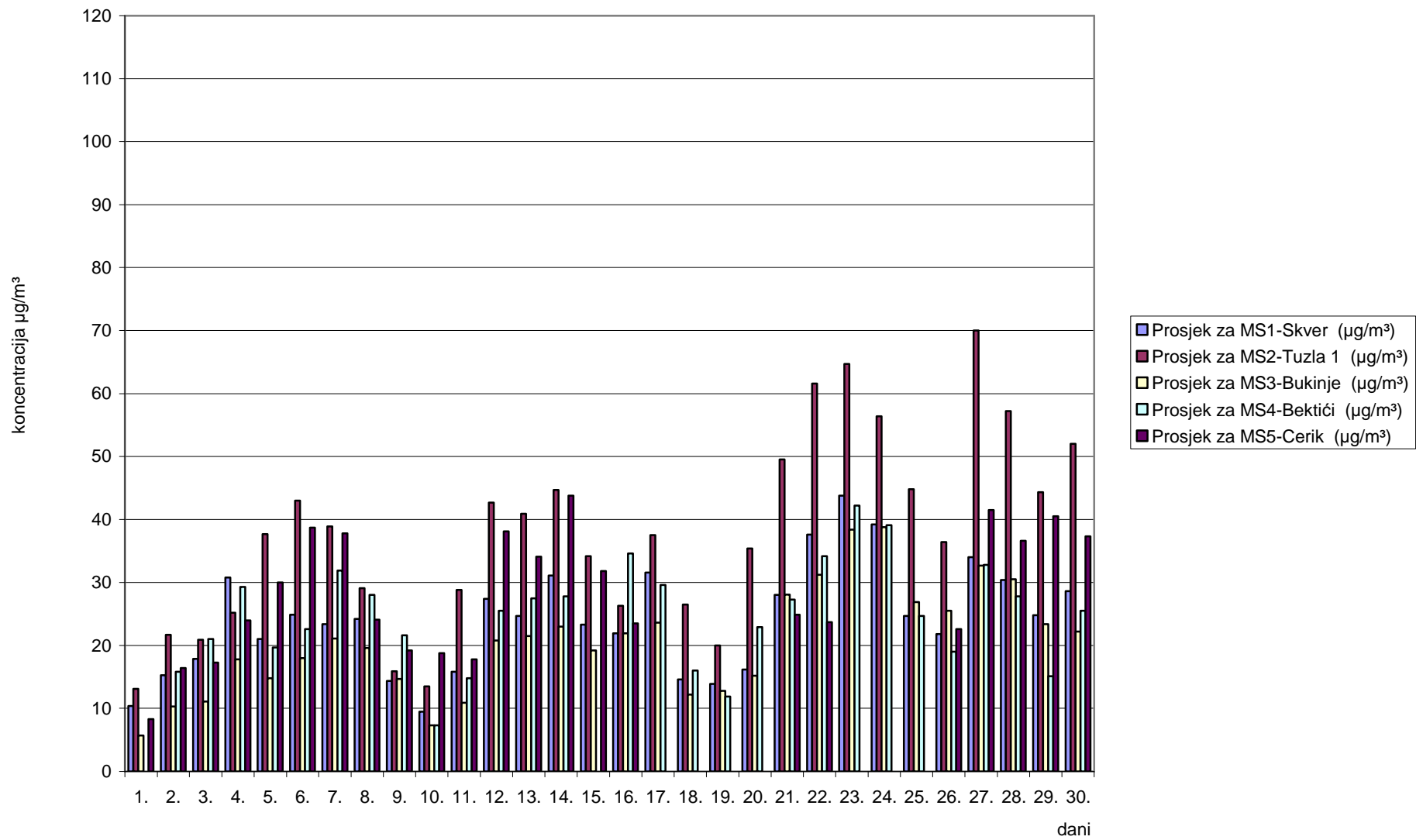
Slika 5. Grafički prikaz prosječnih dnevnih vrijednosti lebdećih čestica (PM 2,5 ) za mjesec septembar/rujan 2010. godine
