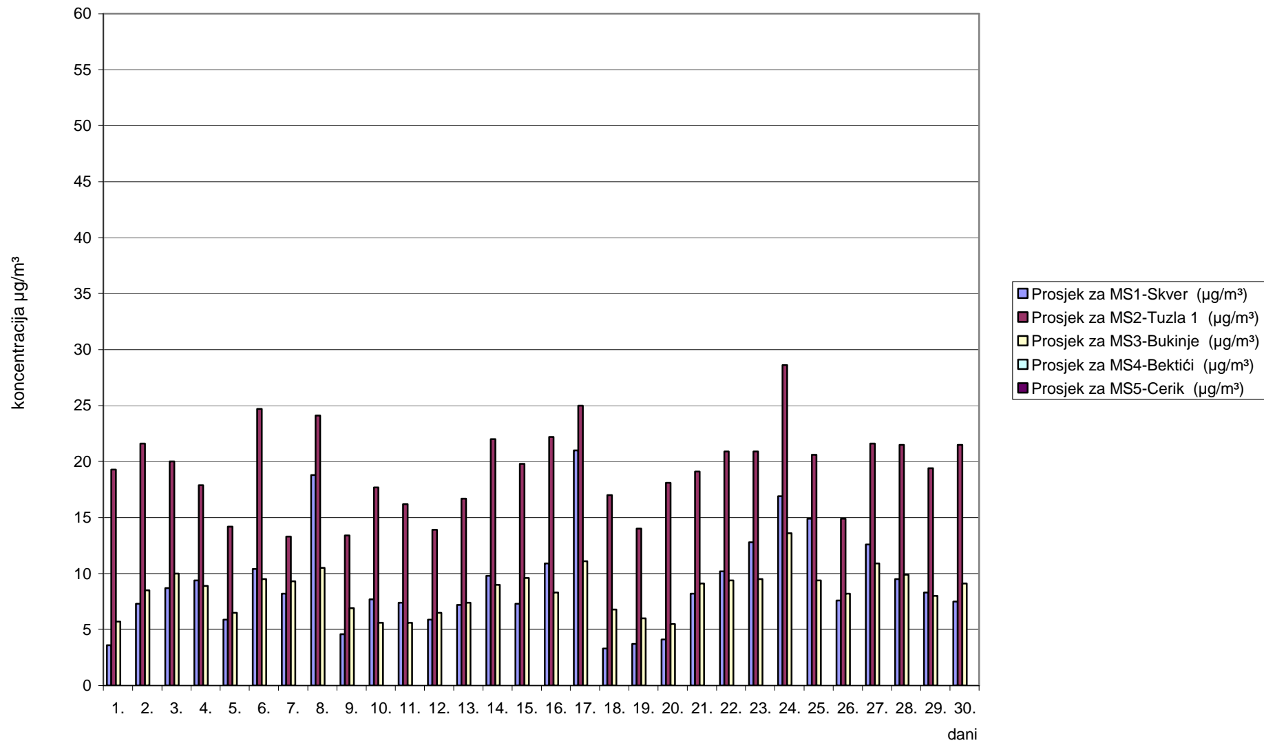
Slika 2. Grafički prikaz prosječnih dnevnih vrijednosti azotdioksida ( \text{NO}_2 ) za mjesec septembar/rujan 2010. godine
