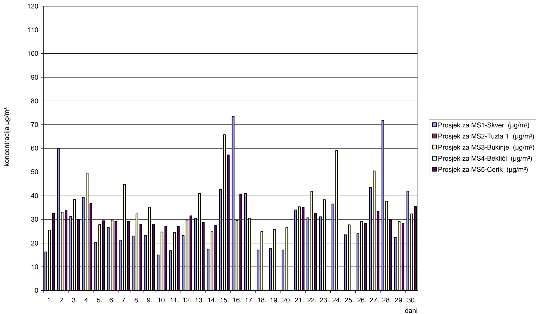
Slika 1. Grafički prikaz prosječnih dnevnih vrijednosti sumpordioksida ( \text{SO}_2 ) za mjesec septembar/rujan 2010. godine
