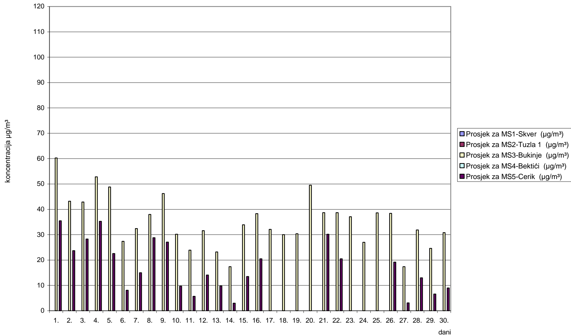
Slika 4. Grafički prikaz prosječnih dnevnih vrijednosti ozona ( \text{O}_3 ) za mjesec septembar/rujan 2010. godine
