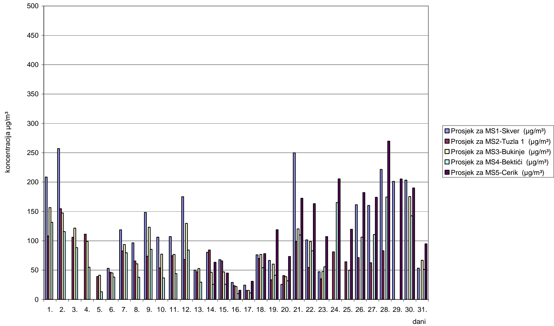
Slika 5. Grafički prikaz prosječnih dnevnih vrijednosti lebdećih čestica (PM 2,5 ) za mjesec decembar/prosinac 2011. godine
