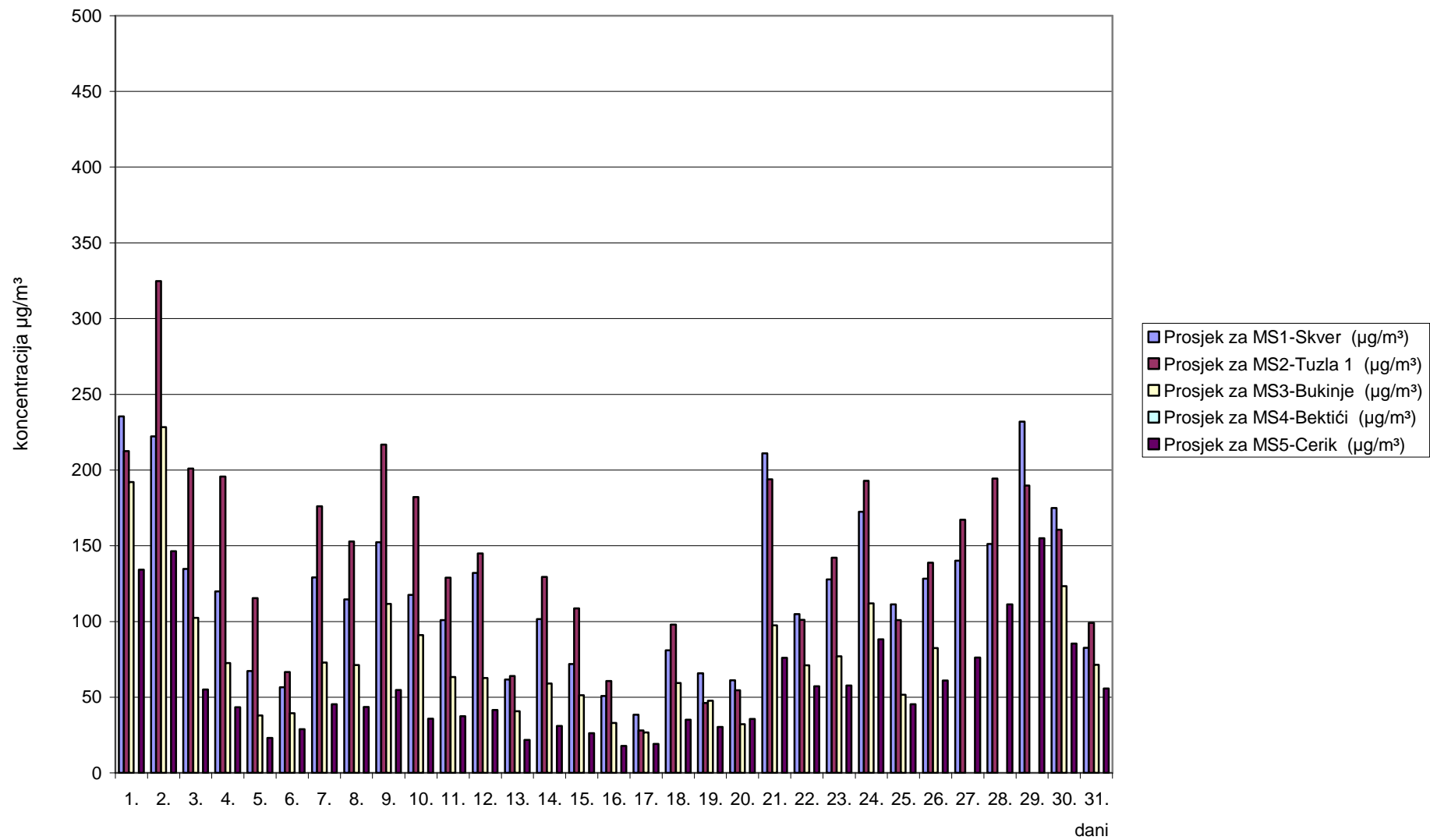
Slika 1. Grafički prikaz prosječnih dnevnih vrijednosti sumpordioksida (SO 2 ) za mjesec decembar/prosinac 2011. godine
