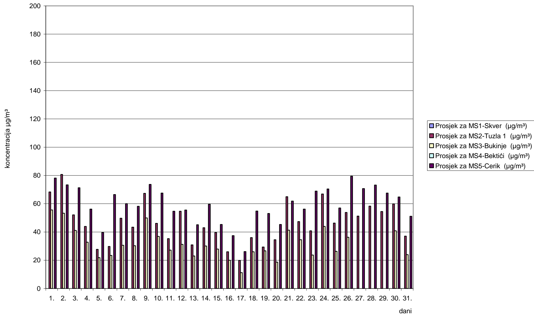
Slika 2. Grafički prikaz prosječnih dnevnih vrijednosti azotdioksida (NO 2 ) za mjesec decembar/prosinac 2011. godine
