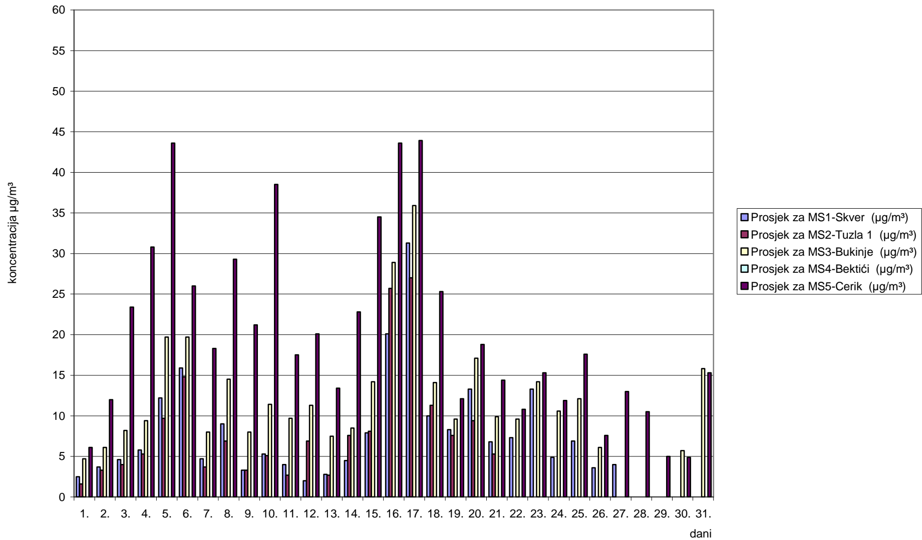
Slika 4. Grafički prikaz prosječnih dnevnih vrijednosti ozona ( \text{O}_3 ) za mjesec decembar/prosinac 2011. godine
