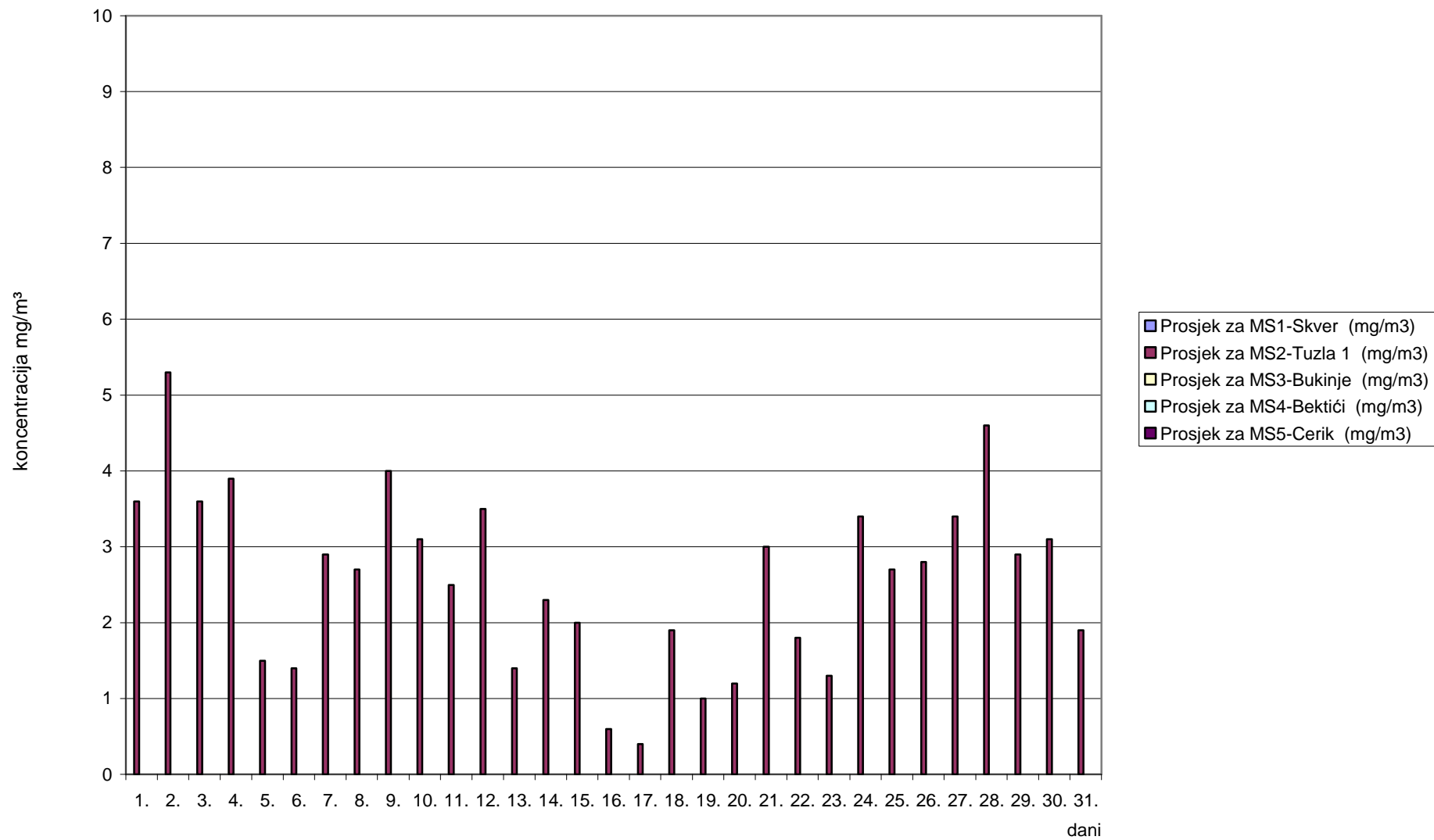
Slika 3. Grafički prikaz prosječnih dnevnih vrijednosti ugljenmonoksida (CO) za mjesec decembar/prosinac 2011. godine
