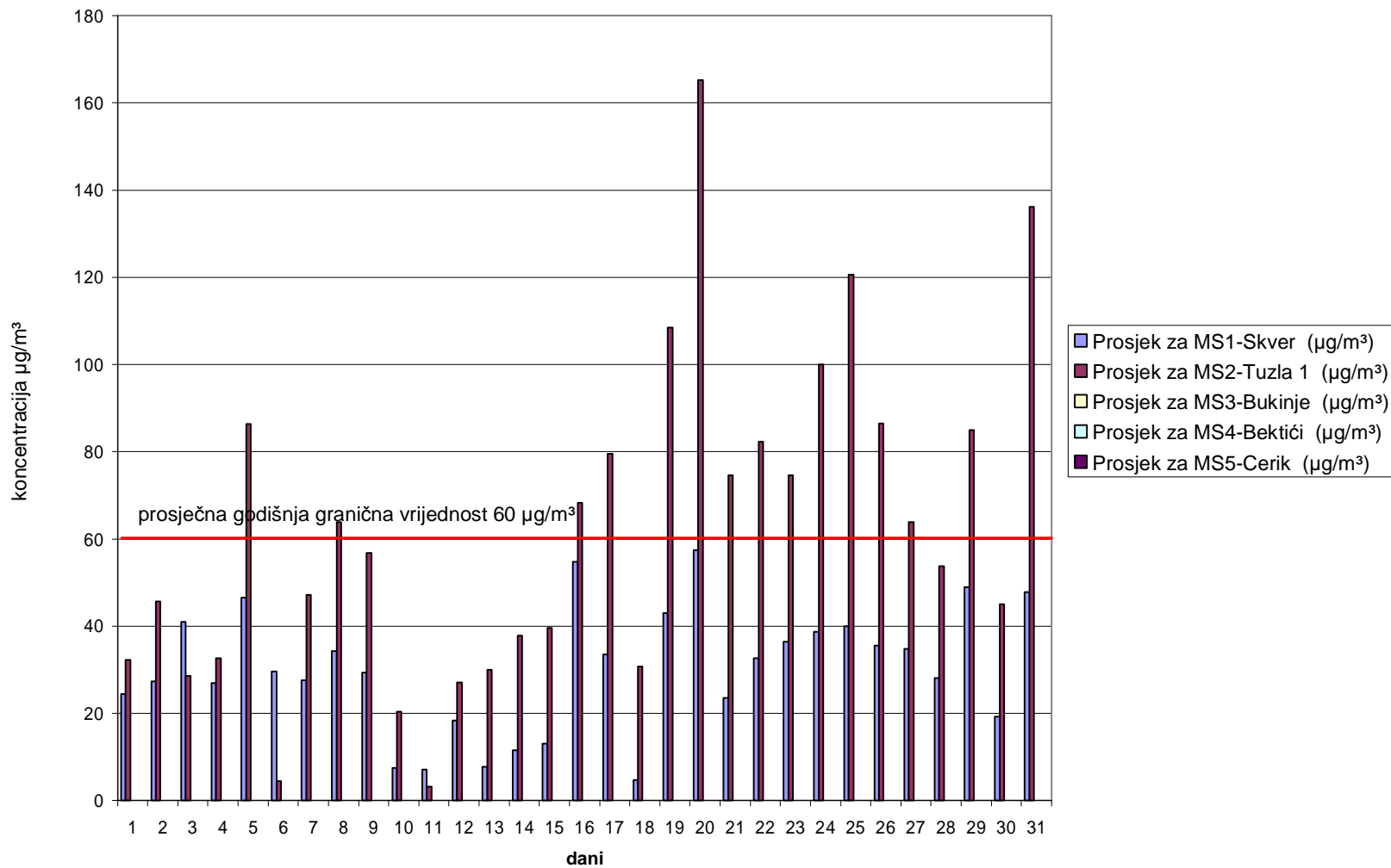
Slika 2. Grafički prikaz prosječnih dnevnih vrijednosti azotdioksida (NO 2 ) za mjesec decembar 2005. godine
