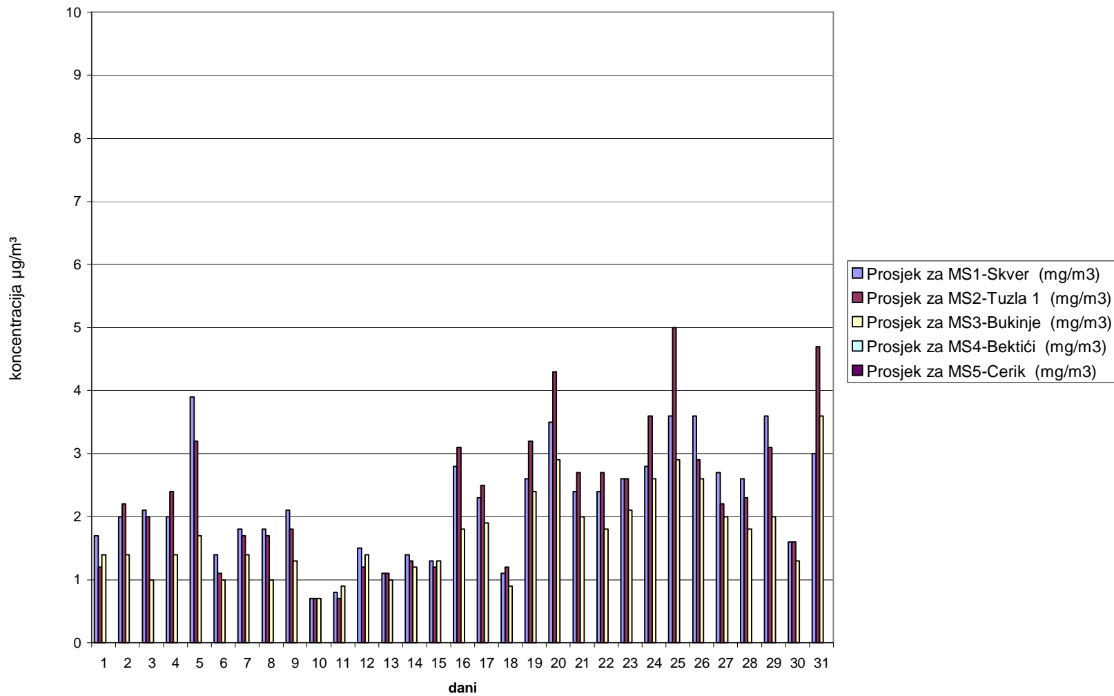
Slika 3. Grafički prikaz prosječnih dnevnih vrijednosti ugljenmonoksida (CO) za mjesec decembar 2005. godine
