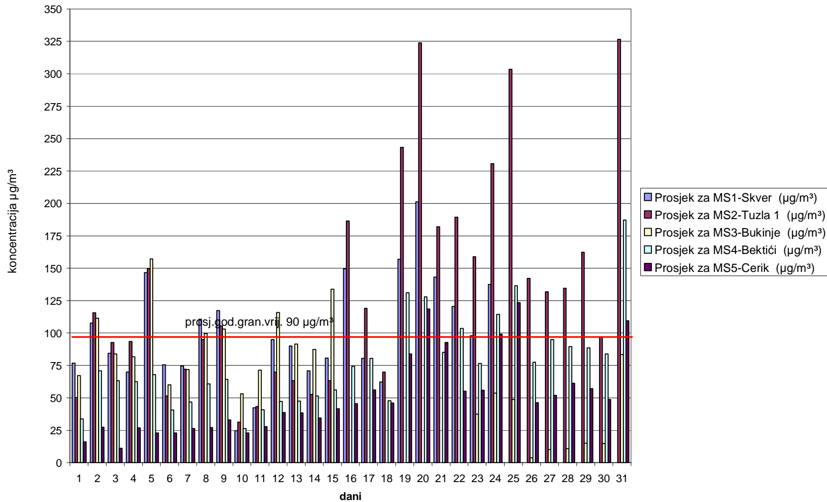
Slika 1. Grafički prikaz prosječnih dnevnih vrijednosti sumpordioksida (SO 2 ) za mjesec decembar 2005. godine
