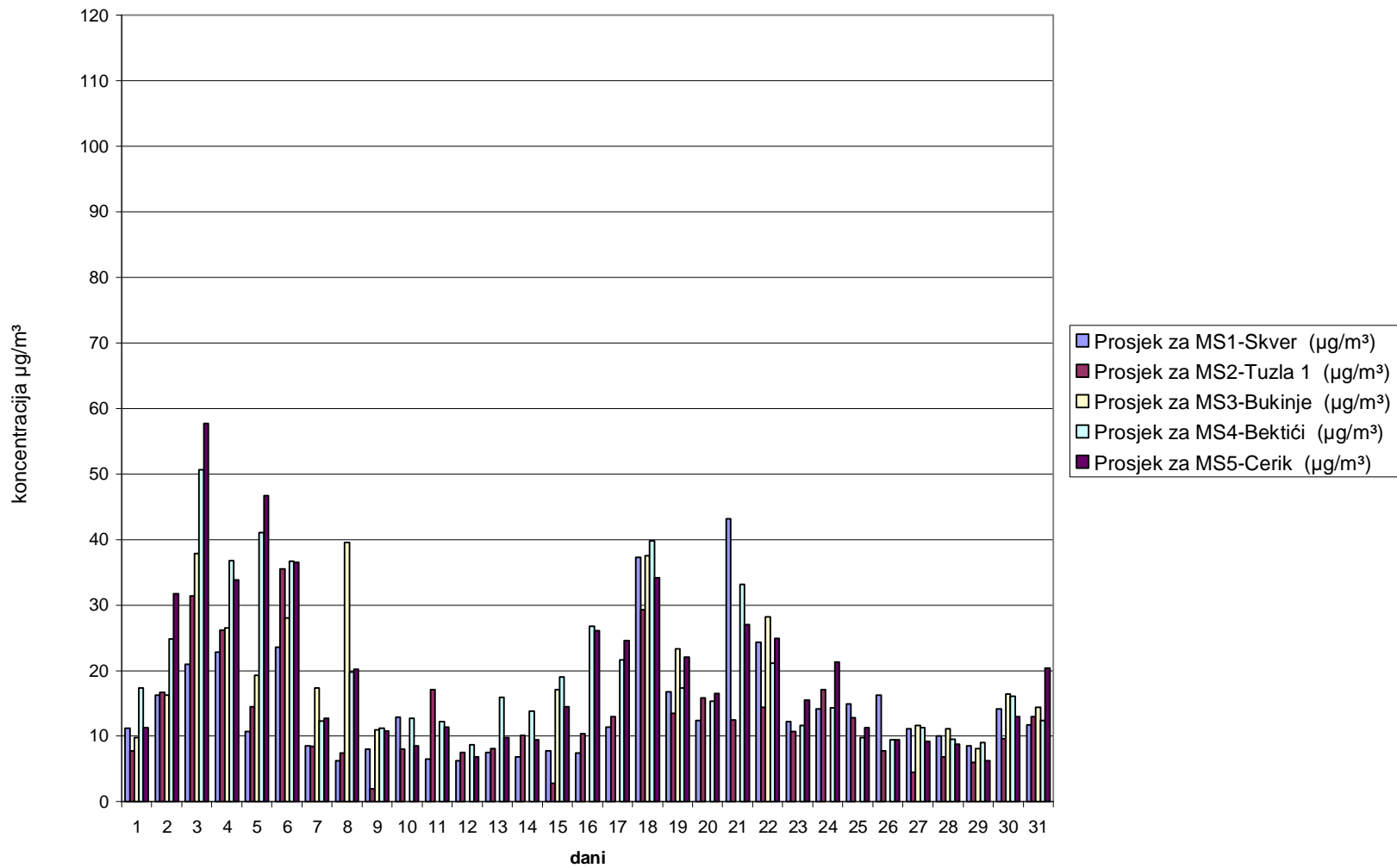
Slika 4. Grafički prikaz prosječnih dnevnih vrijednosti ozona ( O_3 ) za mjesec decembar 2005. godine
