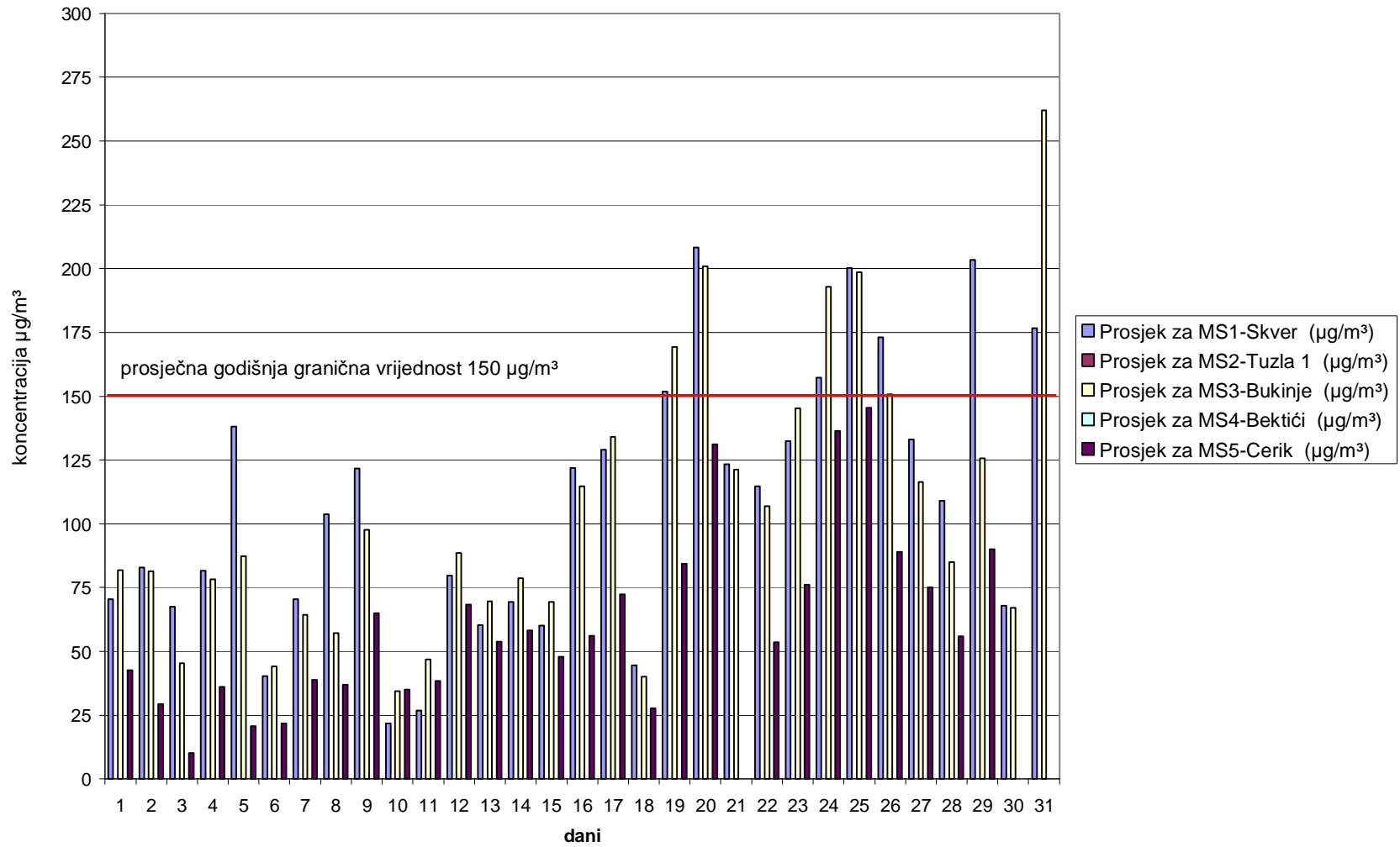
Slika 5. Grafički prikaz prosječnih dnevnih vrijednosti prašine (PM 2,5 ) za mjesec decembar 2005. godine
